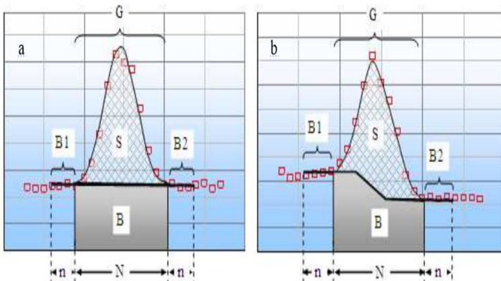
Figure 2.9 – Méthode TPA : B1 et B2 sont le bruit de fond à gauche et à droite du centroïde.
