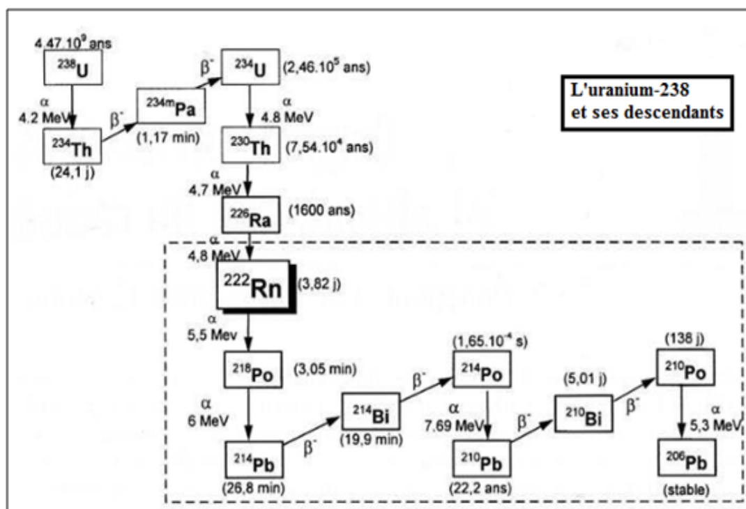
Figure 1.1 – Chaînes de désintégration de ^{238}\text{U} , avec mode de décroissance, énergie émise et demie-vie. Les flèches descendantes montrent l'énergie émise lors de la décroissance \alpha ; Les flèches ascendantes montrent l'énergie émise lors de la décroissance \beta ou \gamma . La zone délimitée par les traits interrompus-courts représente la désintégration du ^{222}\text{Rn} .
