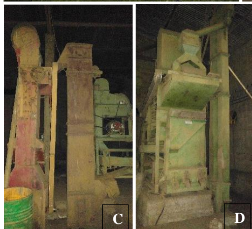
A. visite de l'usine de stockage et de transformation des baies de la COOPAFERLOS ; B. sacs de café stockés depuis environ 2 ans par la coopérative en attendant de potentiels acheteurs ; C et D. machines de dépulpage/décorticage des baies de café.
