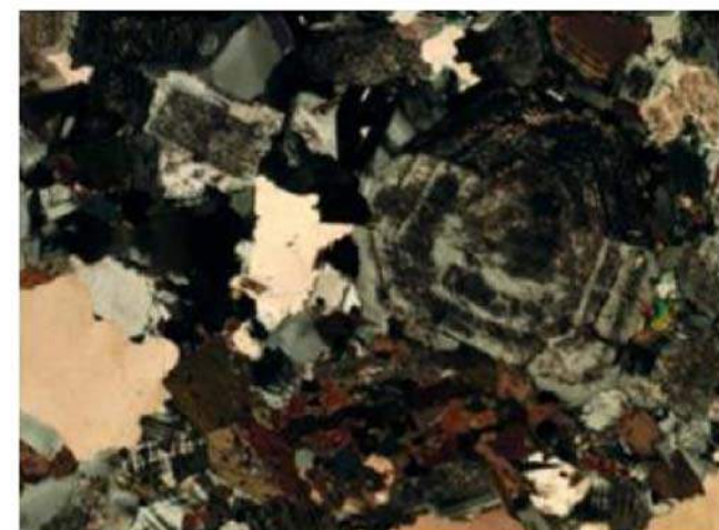
Figure 32. Assemblage minéralogique (Roche d'Aboisso)
