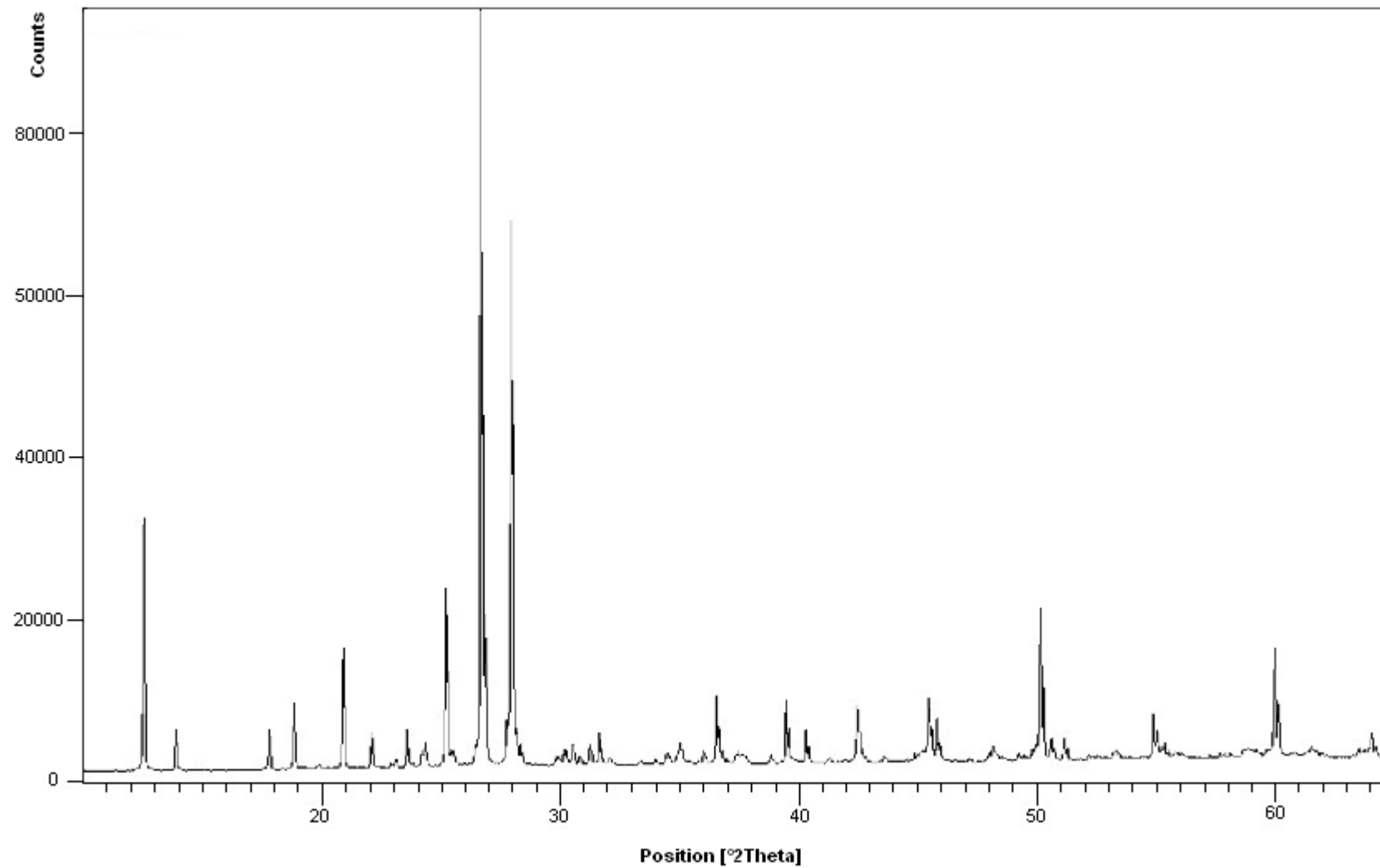
Figure 15. Diffractogramme de la roche de ATTIEKOUA
