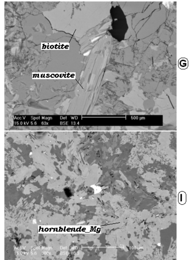
Figure 11. Assemblage des minéraux (image du MEB) Roches de ABIEHOU (G) et de BAKRO (I)
