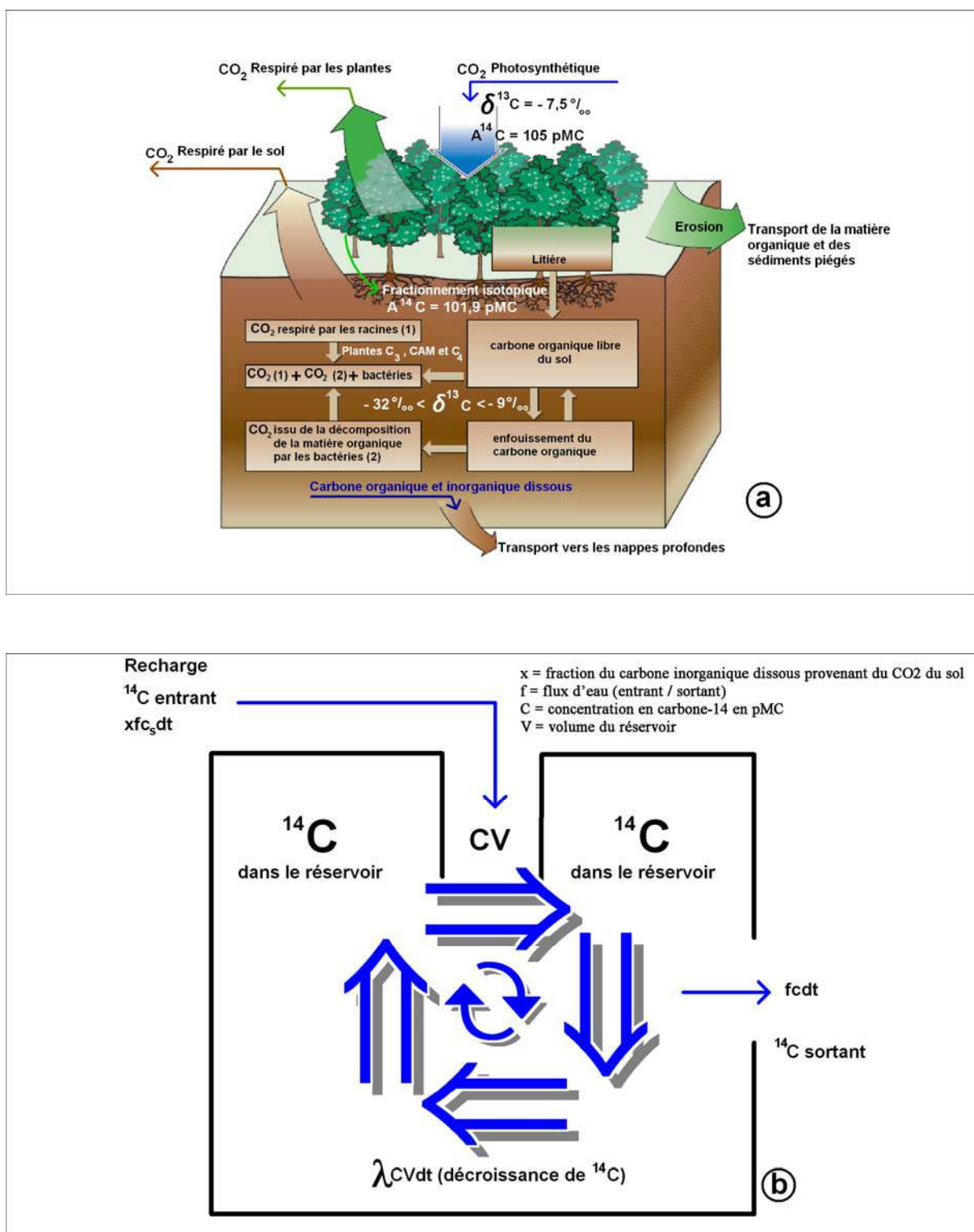
Figure 63. (a) Synthèse du CO 2 du sol de la zone d'étude et (b) Présentation schématique d'un réservoir non stratifié dans le cadre du modèle de mélange parfait
