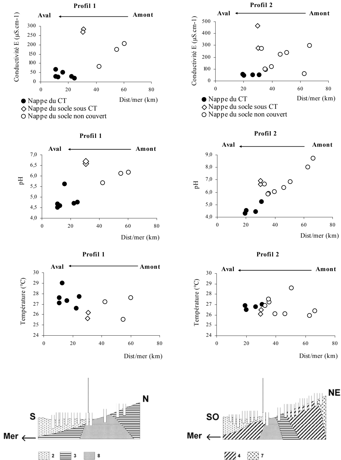
Figure 41. Evolution amont-aval des paramètres physico-chimiques suivant les profils 1 et 2 définis (cf. figure 39)
