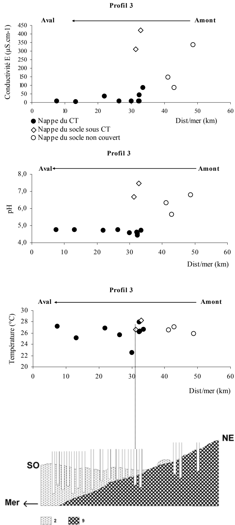
Figure 42. Evolution amont-aval des paramètres physico-chimiques suivant le profil 3 ( cf. figure 39)
