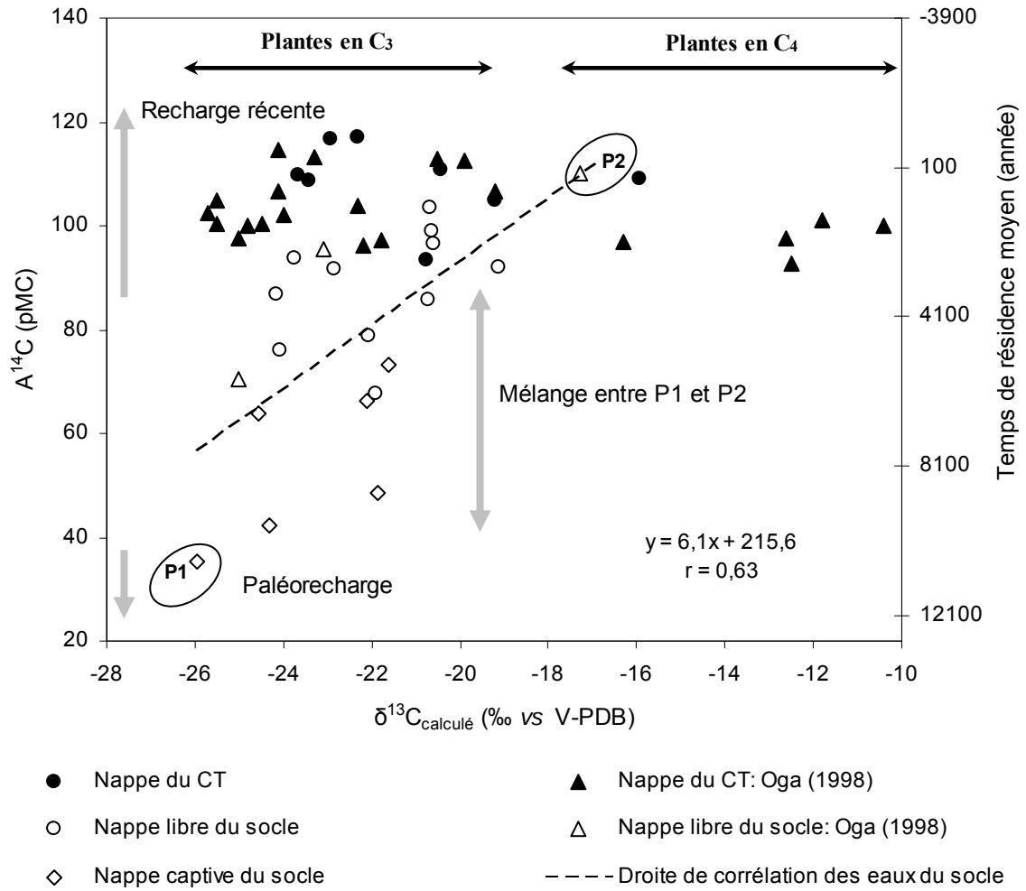
Figure 67. Corrélation entre l'activité en ^{14}C /temps de résidence moyen et la teneur en \delta^{13}C des eaux souterraines étudiées
