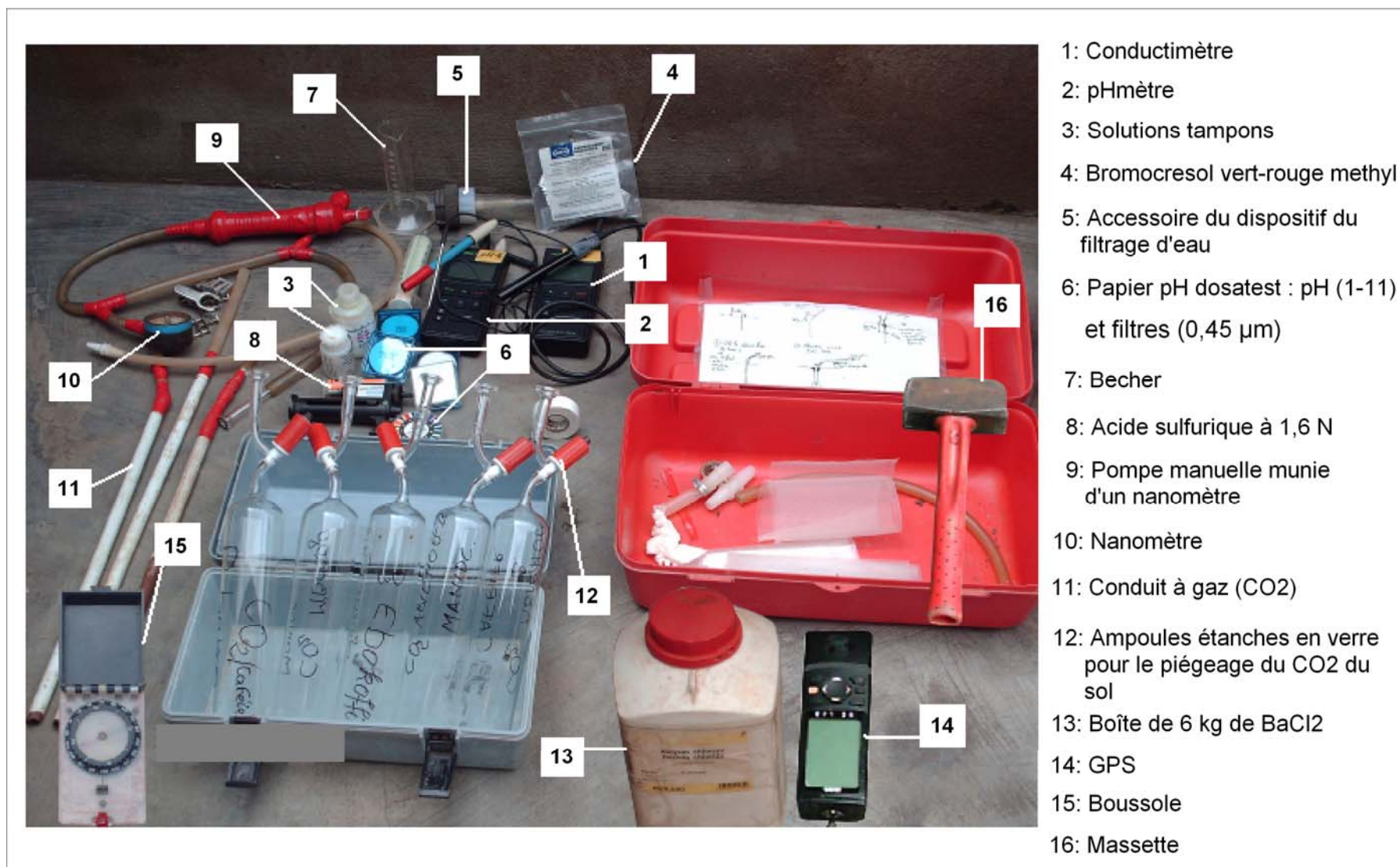
Figure 37. Matériel de terrain
