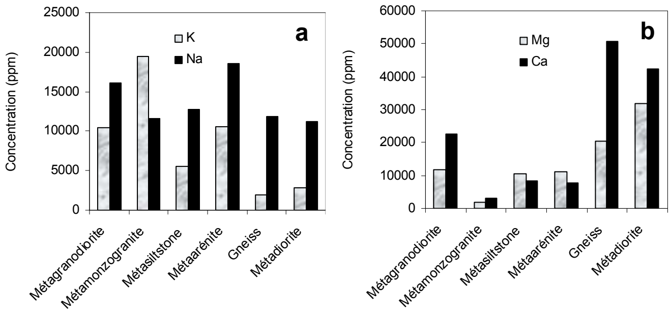
Figure 35. Proportion entre alcalins et entre alcalino-terreux dans chaque type de roche
