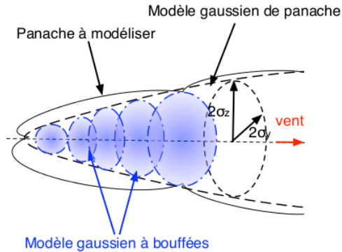
FIGURE 1.11 – Modèle gaussien non stationnaire à bouffées : le panache est discrétisé en une série de bouffées, gaussiennes dans les trois directions.
