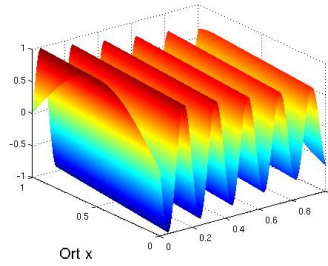
FIGURE 1.16 – simulation sous matlab de l'équation du transport linéaire(advection) avec T=3 , I = [0, 1] , un vent u = 10,4 (voir 1.2), TT(1) = 7000 , XX(1) = 100 : on a toujours la stabilité du schéma.
