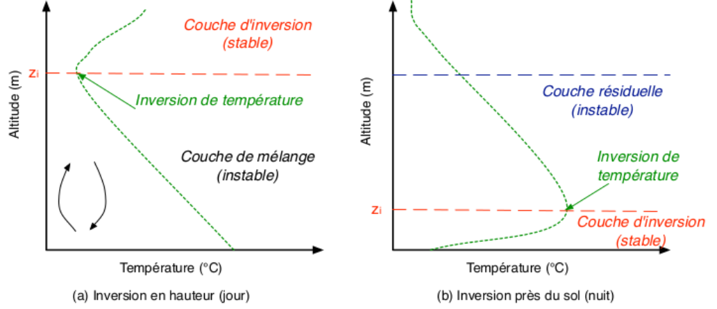
FIGURE 1.10 – Représentation de l'inversion de température dans les deux cas les plus fréquents : (a) inversion en hauteur dans la journée ( z_i de l'ordre de 100 m) et (b) inversion proche du sol la nuit ( z_i de l'ordre de 10 m).
