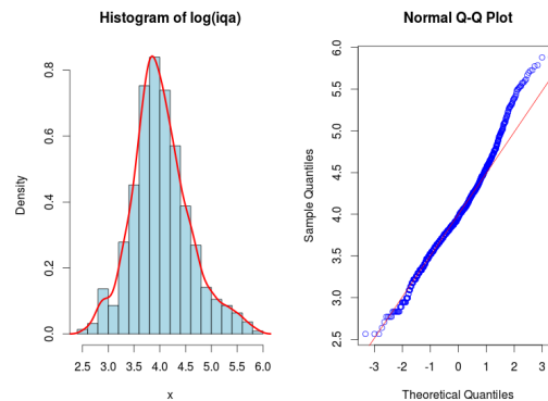
FIGURE 4.7 – Histogramme des résidus et Q - Q plot de \log(iqa) [40]
