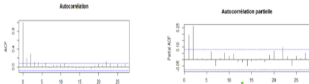
FIGURE 5.1 – ACF et PACF pour la série \log(iqa) .
