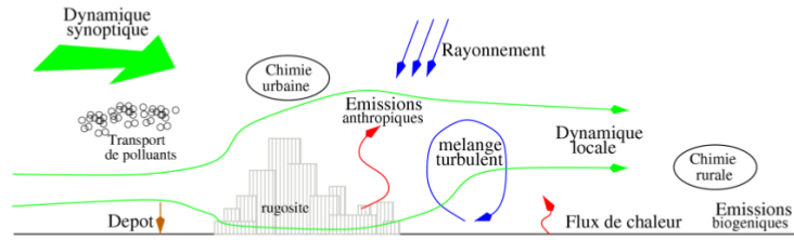
FIGURE 1.4 – Schéma d'un environnement urbain et de tous les processus inter-agissant dans la CLA.
