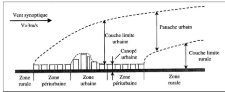
FIGURE 1.5 – Le "panache" urbain : structure verticale de l'atmosphère urbaine pour des vents supérieurs à 3m/s (Ringenbach (2004), d'après Mestayer et Anquetin (1995)).
