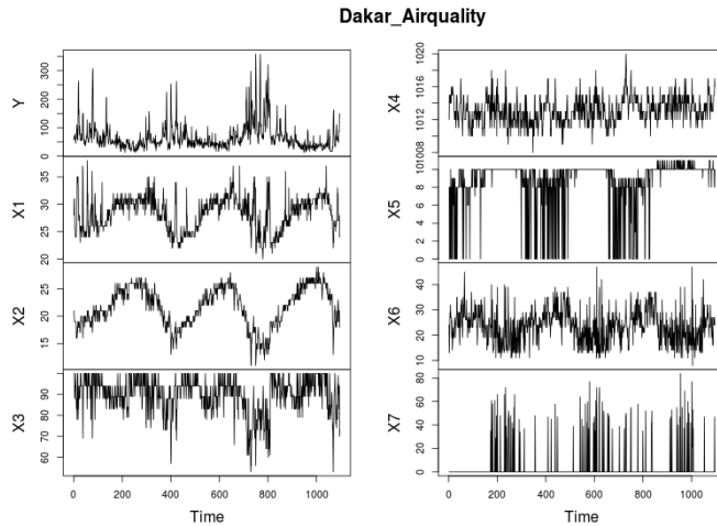
FIGURE 4.5 – Courbes des différentes séries temporelles.
