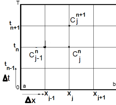
FIGURE 1.13 – Domaine de discrétisation
