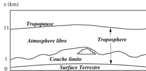
FIGURE 1.3 – Coupe verticale de la basse atmosphère
