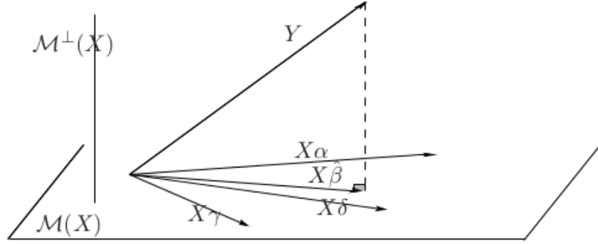
FIGURE 4.6 – Représentation de \hat{X}\beta dans l'espace des variables.
