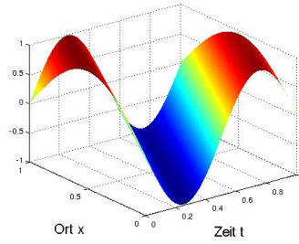
FIGURE 1.14 – simulation sous matlab de l'équation du transport linéaire (advection) avec T=1 , I = [0, 1] , un vent de vitesse u = 2 , \Delta x = 0,01 , \Delta t = 0,00142 , \sigma = 0,284 \leq 1 : on a la stabilité du schéma
