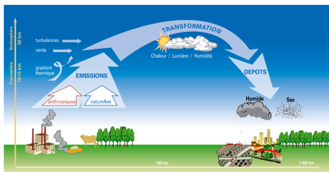
FIGURE 1.1 – Illustration de la dispersion atmosphérique. Source : ADEME
