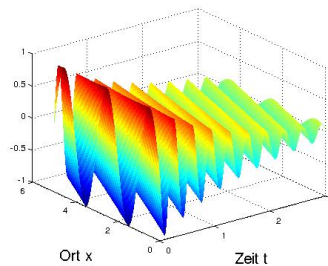
FIGURE 1.17 – simulation sous matlab de l'équation du transport linéaire(advection) avec T=3 , I = [0, 5] , un vent u = 6 , TT(1) = 700 , XX(1) = 100 , \sigma > 1 : on a un schéma instable
