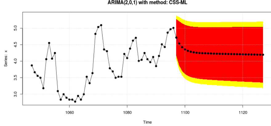
FIGURE 5.2 – Prévisions et intervalle de confiance à 90% en rouge et 95% en jaune.
