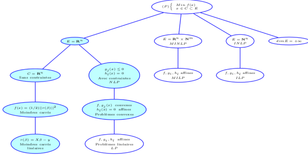
FIGURE 3.1 – Classification des problèmes d'optimisation.
