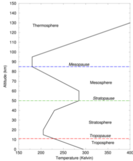
FIGURE 1.2 – Description schématique de la structure verticale de l'atmosphère
