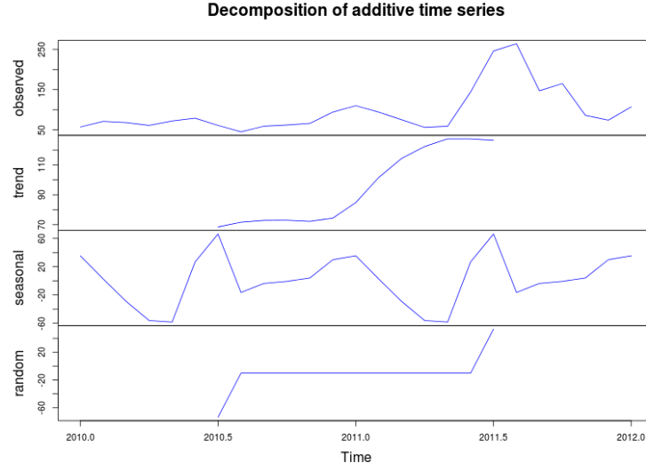
FIGURE 4.2 – Décomposition additive de la série indice de la qualité de l'air (iqa) à Dakar : période 2010 à 2012
