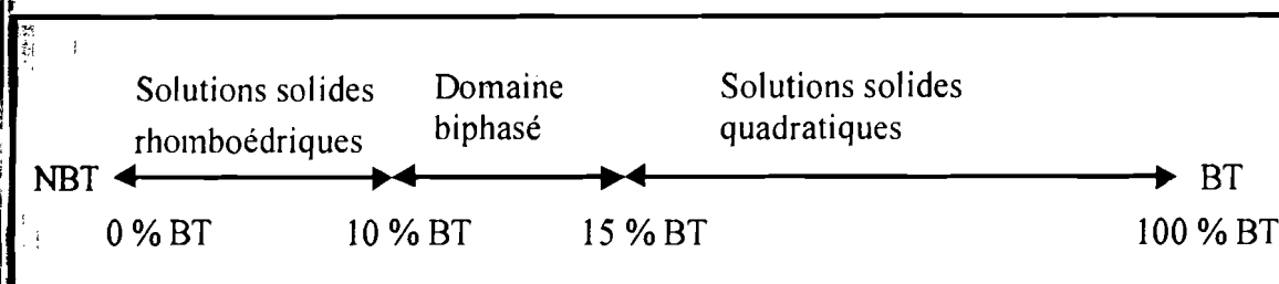
Fig. II.3 : Domaines d'existence des solutions solides du système (1-x) NBT - x BT.
