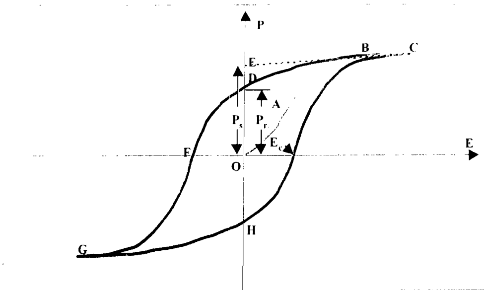
Fig.1.3 Cycle d'hystérésis des cristaux ferroélectriques.
