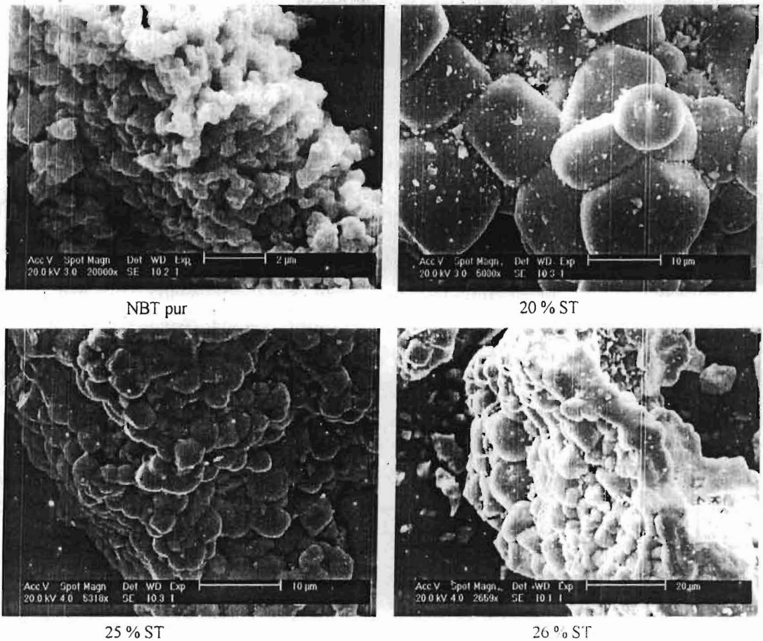
Fig.II.23. : Microstructure de quelques compositions du système (1 - x)\text{NBT} - x\text{ST}
