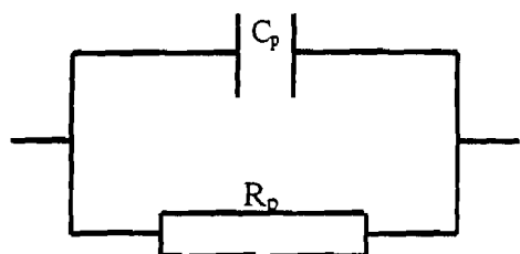
Fig.III.2. : Circuit équivalent
