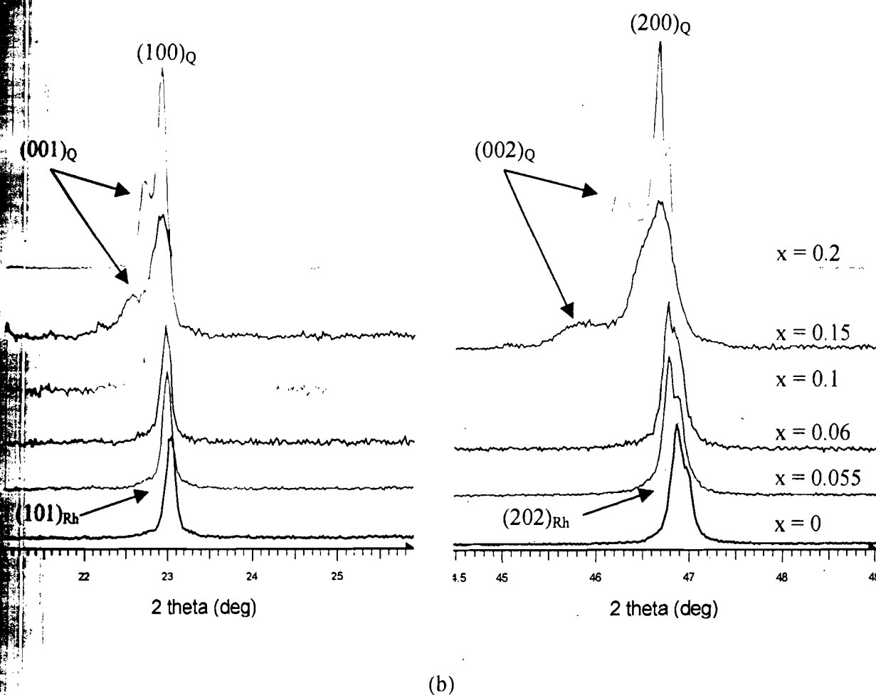
Fig. II.2 : Diagrammes de diffraction des rayons X des solutions solides à température ambiante.
