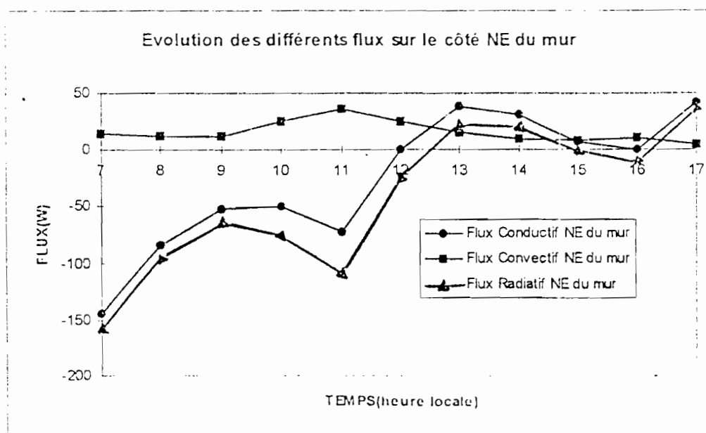
FIGURE.4.6.d: Etude comparative des différents flux sur le côté NE du mur
