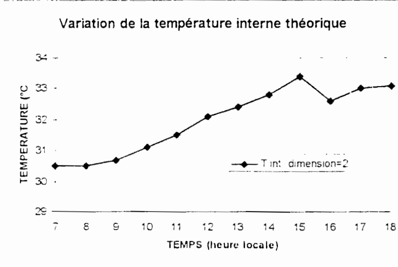
FIGURE.4.2.b: Evolution temporelle de la température interne
