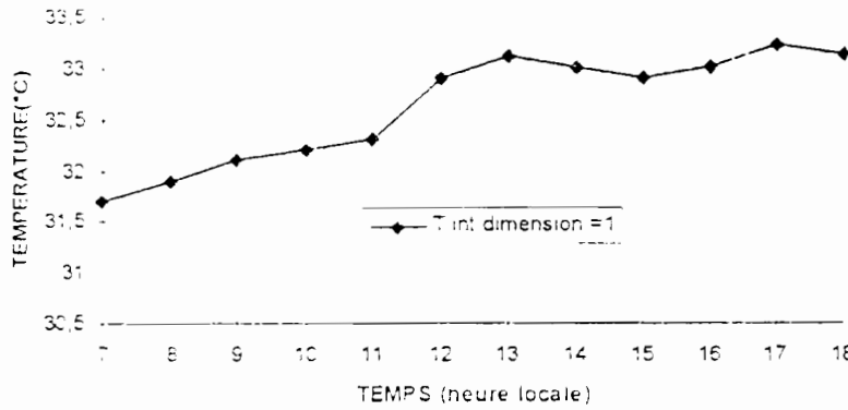
Variation de la température interne théorique
