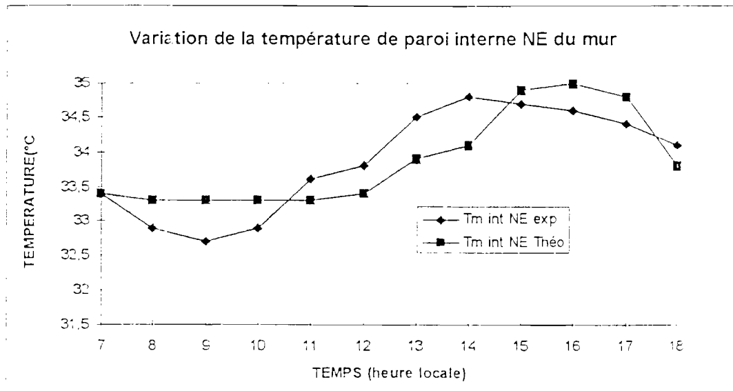
FIGURE.4.3.a-7: Comparaison courbes théorique et expérimentale
