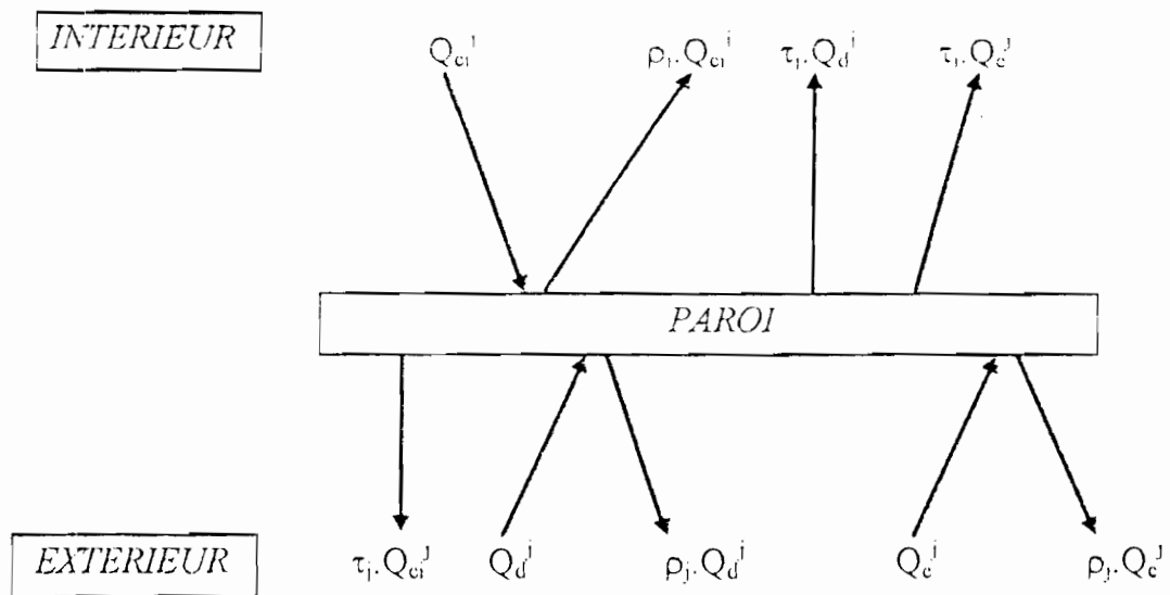
FIGURE.3.7 : Schématisation des différents échanges radiatifs
