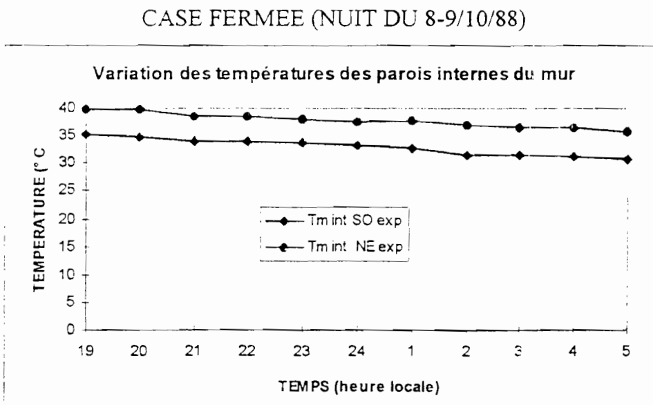
FIGURE.2.5.c.2: Evolution des températures des parois internes du mur
