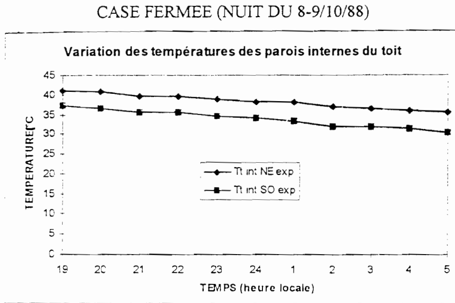
FIGURE.2.5.c.1: Evolution des températures des parois internes du toit
