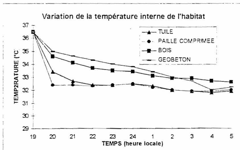
FIGURE.4.11.c Evolution de la température interne en fonction des matériaux locaux
