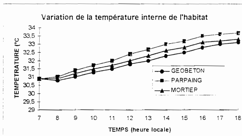
FIGURE.4.11.b Evolution de la température interne en fonction des matériaux (gébéton et matériaux modernes)
