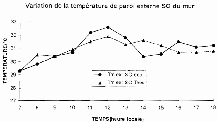
FIGURE.4.4.a-6: Comparaison courbes théorique et expérimentale
