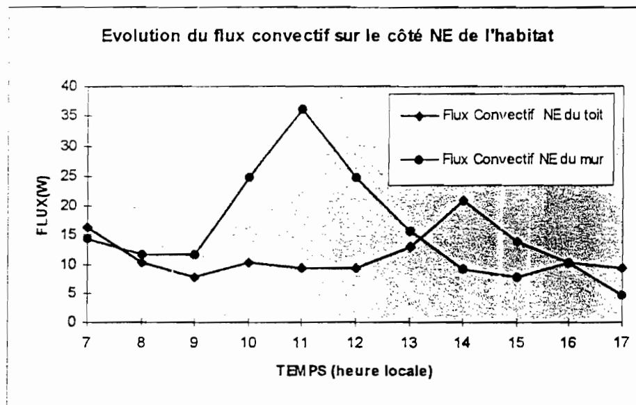
FIGURE.4.8.b:Etude comparative des flux convectifs sur le côté NE de l'habitat
