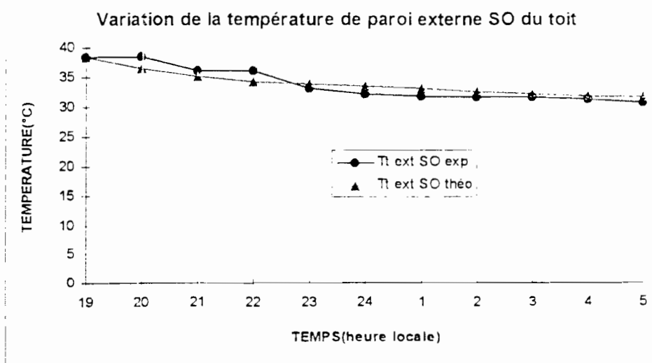
FIGURE.4.3.c-4: Comparaison courbes théorique et expérimentale
