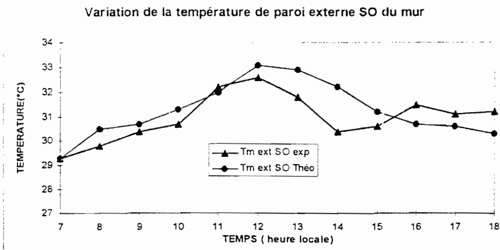
FIGURE.4.3.a-6: Comparaison courbes théorique et expérimentale
