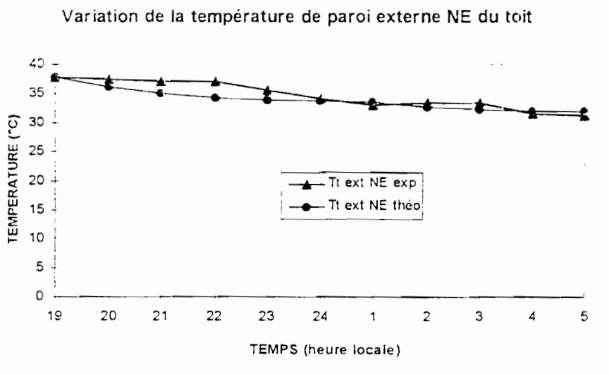
FIGURE.4.3.c-2: Comparaison courbes théorique et expérimentale
