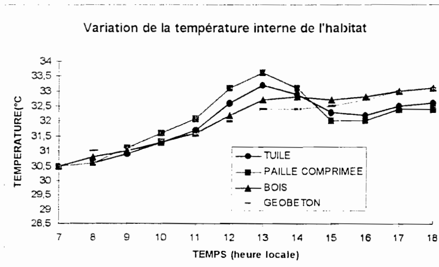
FIGURE.4.12.a Evolution de la température interne en fonction des matériaux locaux
