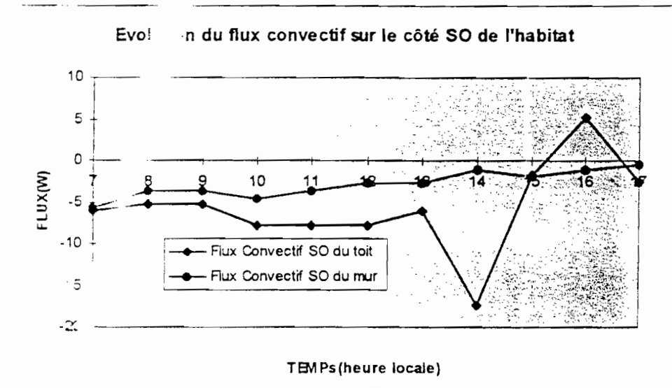
FIGURE.4.8.a:Etude comparative des flux convectifs sur le côté SO de l'habitat
