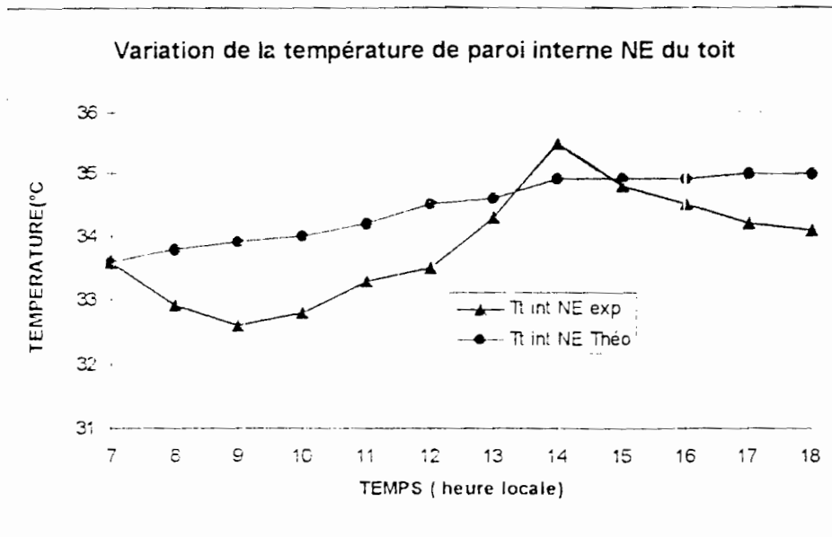
FIGURE.4.3.a-1: Comparaison courbes théorique et expérimentale
