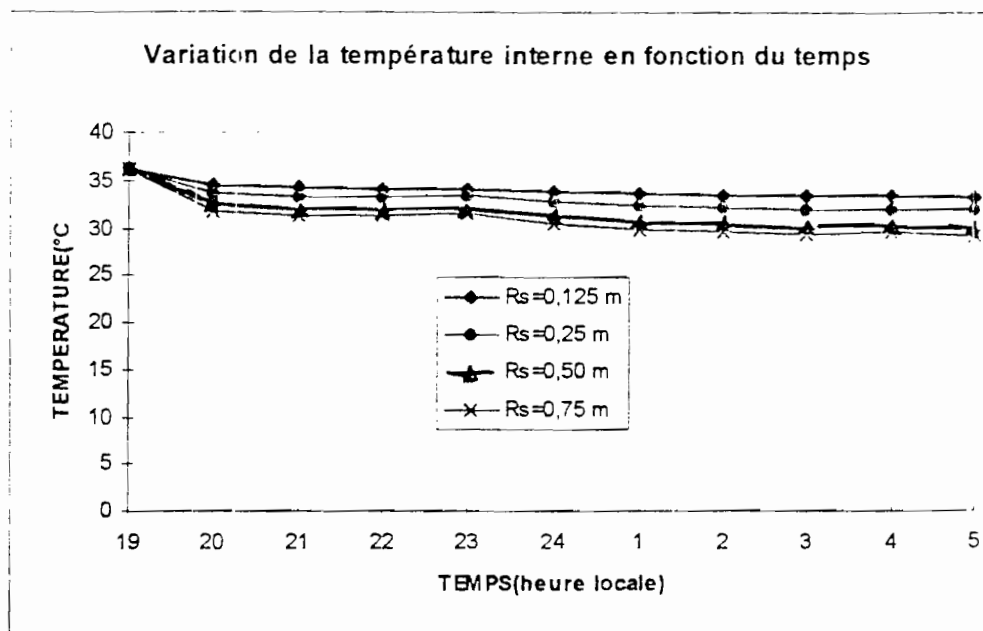
FIGURE.4.9.c Evolution de la température interne en fonction de l'ouverture
