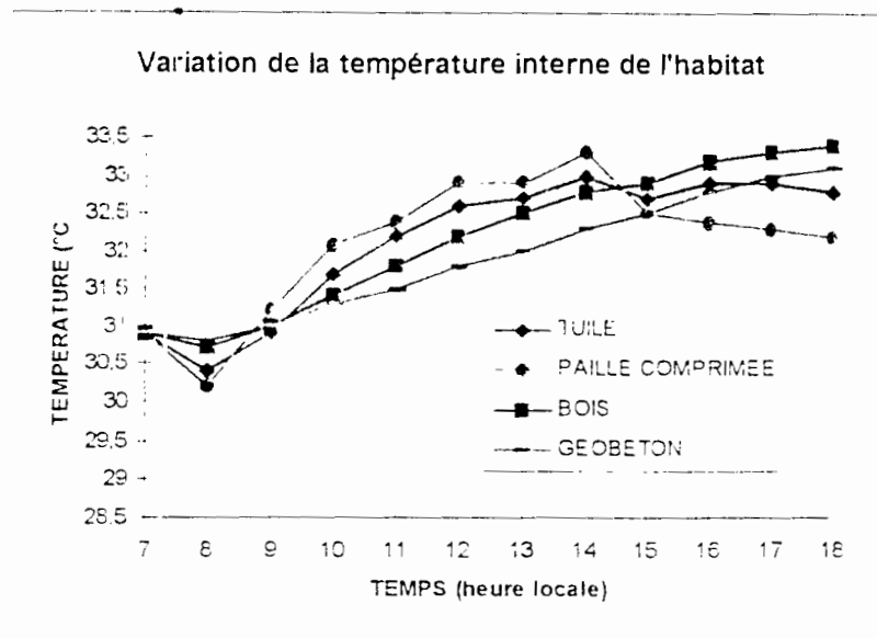
FIGURE.4.12.b Evolution de la température interne en fonction des matériaux locaux
