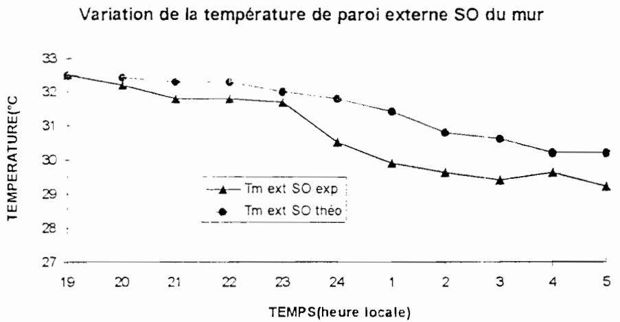
FIGURE.4.4.c-6: Comparaison courbes théorique et expérimentale
