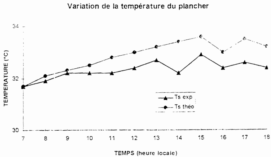
FIGURE.4.4.b-9: Comparaison courbes théorique et expérimentale
