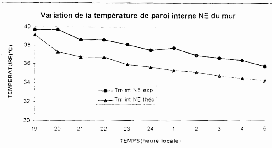
FIGURE.4.4.c-7: Comparaison courbes théorique et expérimentale
