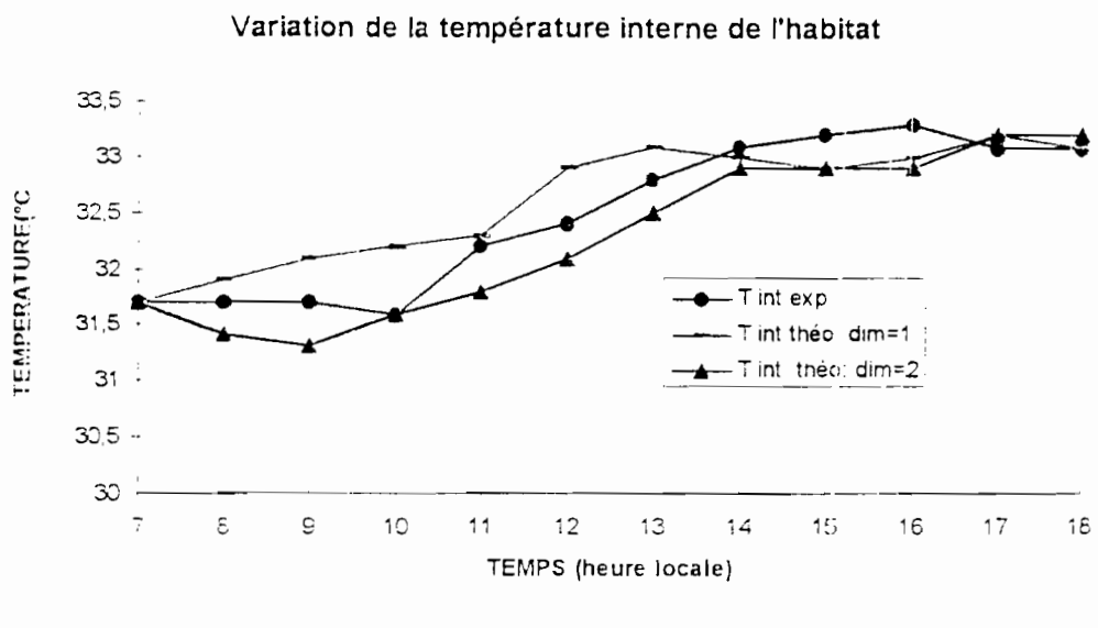
FIGURE.4.5.a: Comparaison température unidimensionnelle et bidimensionnelle
