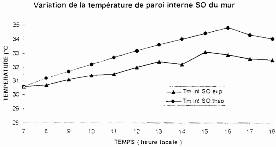
FIGURE.4.3.b-5: Comparaison courbes théorique et expérimentale
