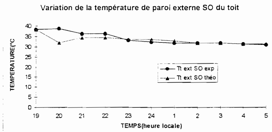
FIGURE.4.4.c-2: Comparaison courbes théorique et expérimentale
