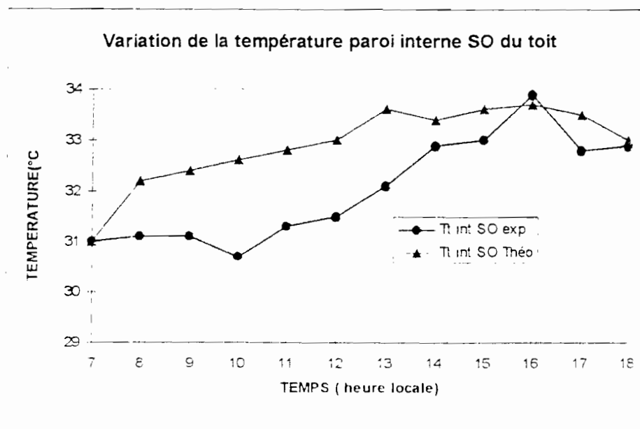
FIGURE.4.3.a-3: Comparaison courbes théorique et expérimentale
