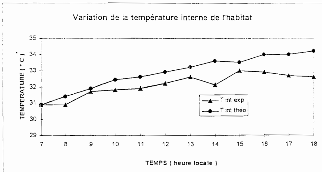
FIGURE.4.3.b-8: Comparaison courbes théorique et expérimentale
