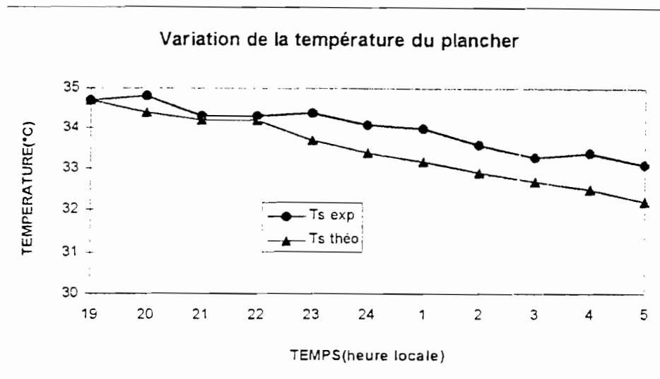
FIGURE.4.4.c-9: Comparaison courbes théorique et expérimentale
