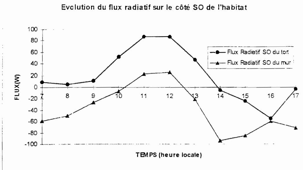
FIGURE.4.7.b:Etude comparative des radiatifs sur le côté SO de l'habitat
