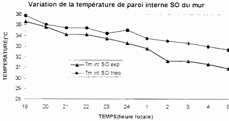
FIGURE.4.4.c-5: Comparaison courbes théorique et expérimentale
