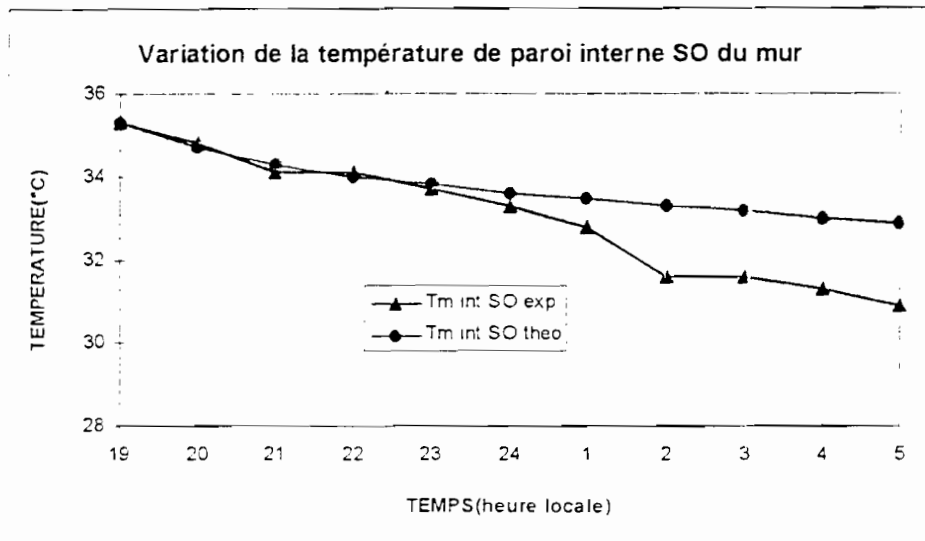
FIGURE.4.3.c-5: Comparaison courbes théorique et expérimentale
