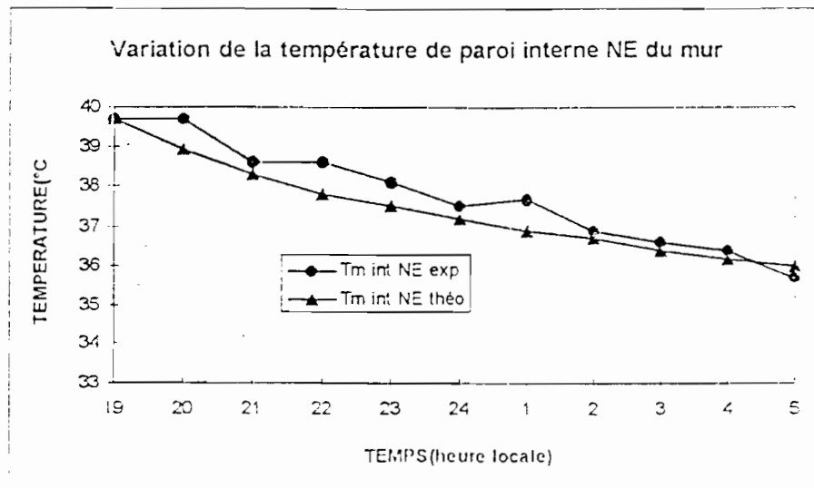
FIGURE.4.3.c-7: Comparaison courbes théorique et expérimentale
