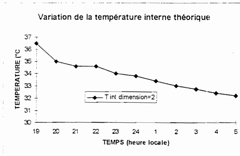
FIGURE.4.2.c: Evolution temporelle de la température interne
