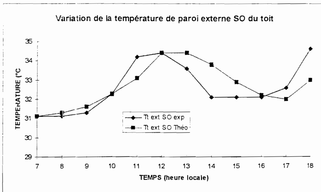
FIGURE.4.3.a-4: Comparaison courbes théorique et expérimentale
