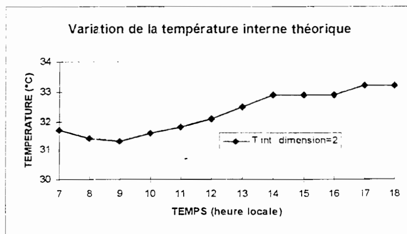
FIGURE.4.2.a: Evolution temporelle de la température interne
