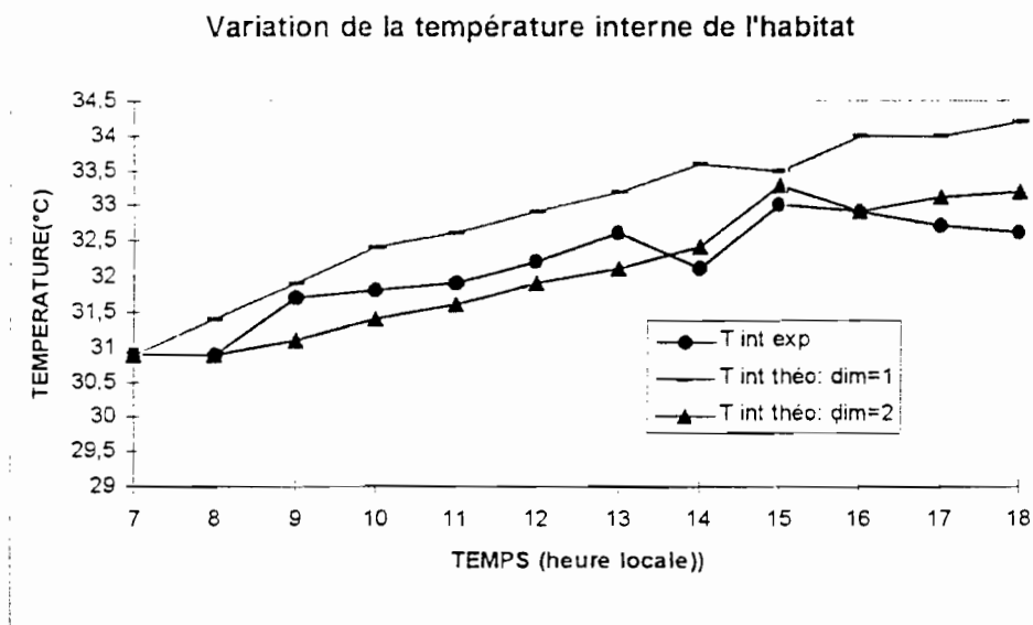
FIGURE.4.5.b: Comparaison température unidimensionnelle et bidimensionnelle
