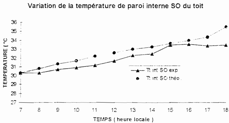
FIGURE.4.3.b-3: Comparaison courbes théorique et expérimentale
