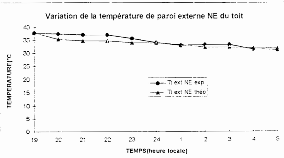
FIGURE.4.4.c-4: Comparaison courbes théorique et expérimentale
