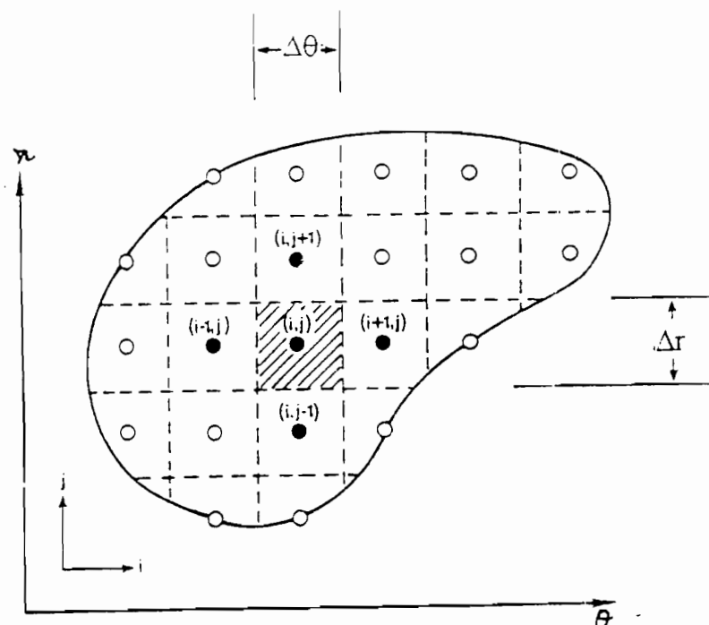
FIGURE.316: représentation d'un élément de volume interne au maillage{28}
