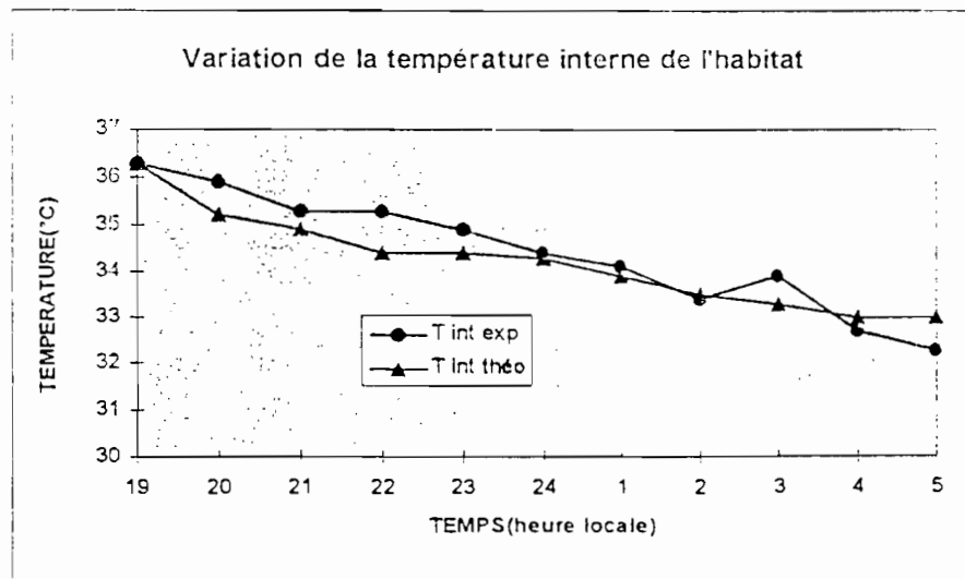
FIGURE.4.3.c-8: Comparaison courbes théorique et expérimentale
