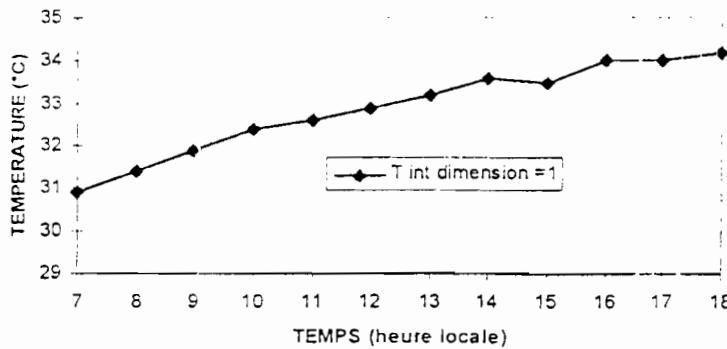
Variation de la température interne théorique
