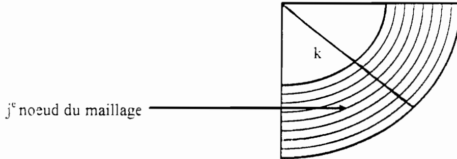
FIGURE.3.13 : Maillage unidimensionnel d'un secteur angulaire ( k )
