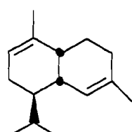
\delta -muurolène 13
