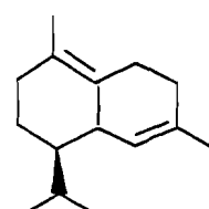
\delta -cadinène 15
