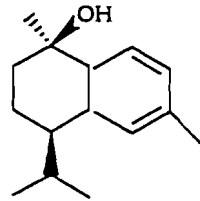
cadinadiénol-I 66
