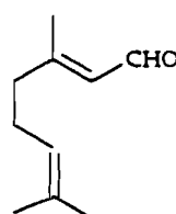
gérانيا1 7
