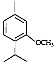
méthyl-thymyléther 62
