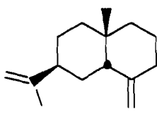
\beta -séliène 14
