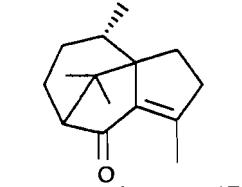
patchoulénone 47
