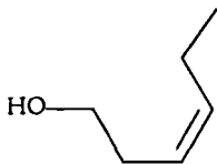
hex-3-énoL-Z 94
