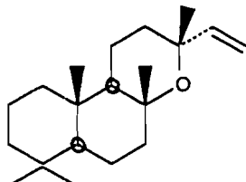
viridiflorène 69
