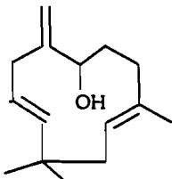
humulénol-II 65
