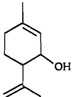
carvéol 61
