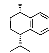
cis-calaménène 16
