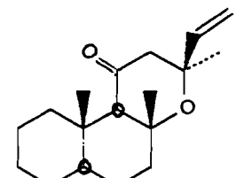
β-bourbonène 72
