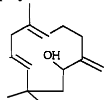
humulénol-I 64
