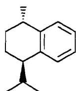
trans-calaménène 17
