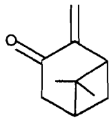
pinocarvone 58
