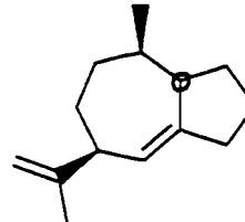
δ-guaiène 63
