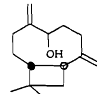
caryophylladiénol 24
