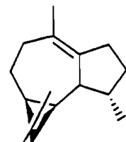
viridiflorène 69
