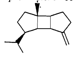
β-bourbonène 72
