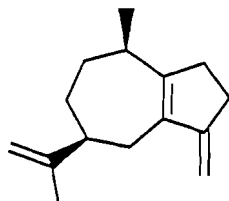
guaiatriène 70
