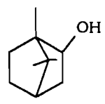
bornéol 110
