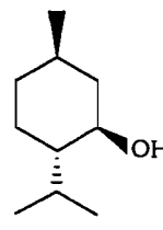
menthol 96
