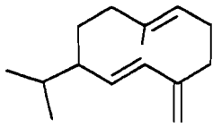
germacrène D 57
