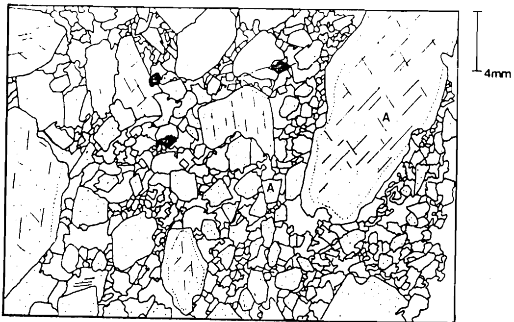
Fig. 28 - Texture des gabbros à mégacrists d'amphibole dans la partie méridionale de la série de Tonkouto. L'amphibole (A), dont la taille peut dépasser 1 cm, est zonée.
