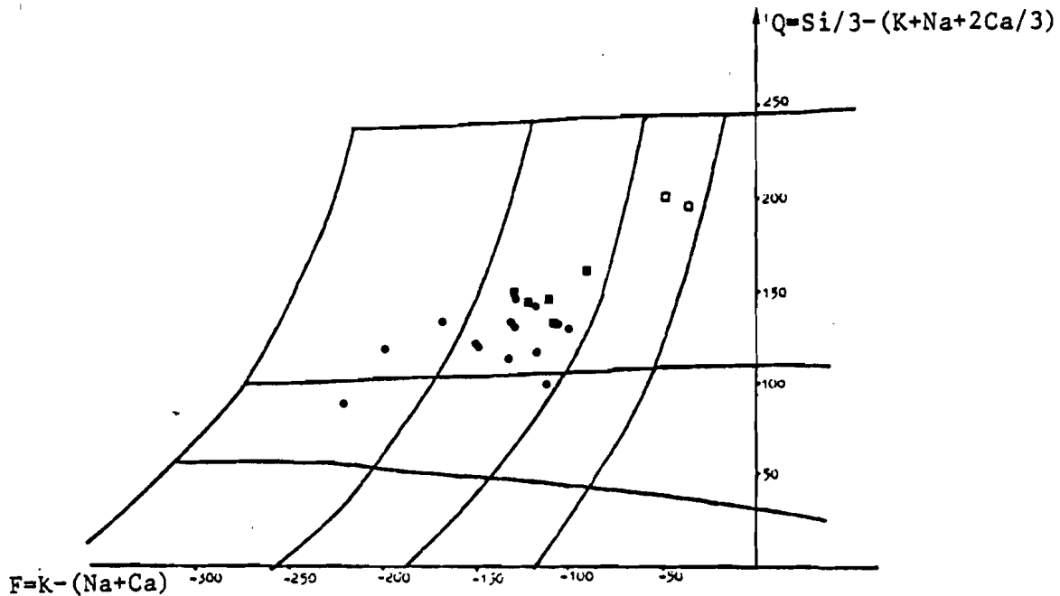
Fig. 69b- Distribution des granitoïdes dans le diagramme Q-F (de la Roche 1964); (légende identique à celle de la figure 69a).
