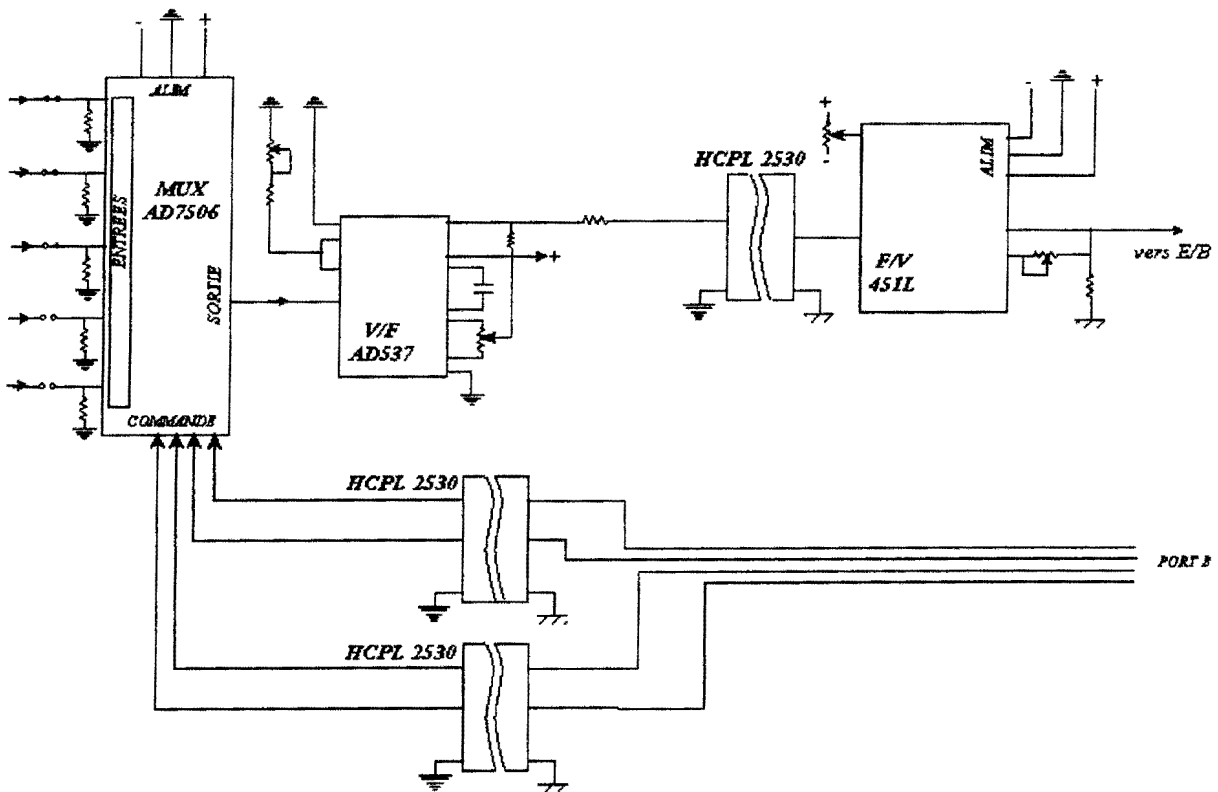
Figure 3. 7: Multiplexage et isolation galvanique
