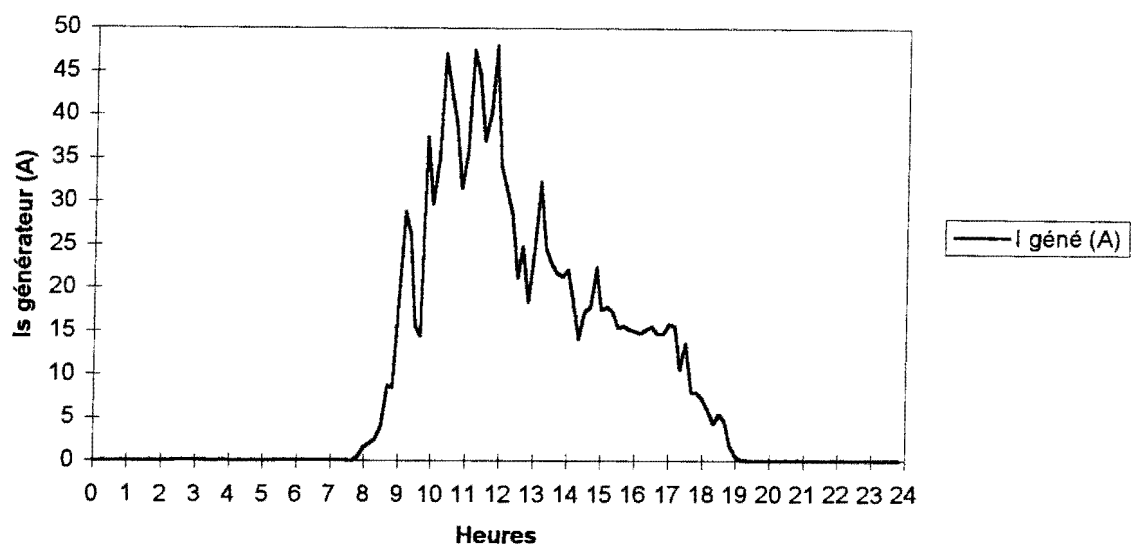
Figure 5. 17: Evolution du courant de sortie du générateur
