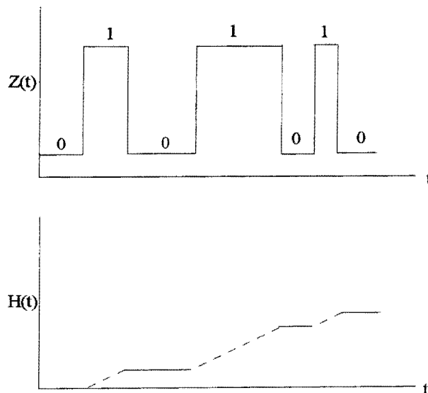
Figure 2. 8: Fonction Z(t) des événements ERC et fonction H(t) de DARC
