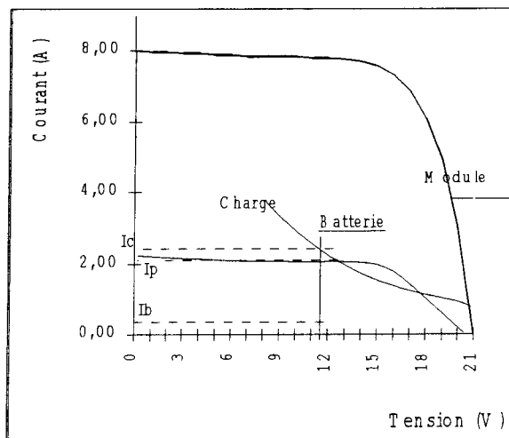
Figure 1.32: Déconnexion partielle du générateur
