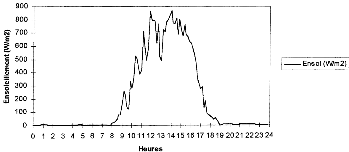
Figure 5. 13: Evolution journalière de l'ensoleillement
