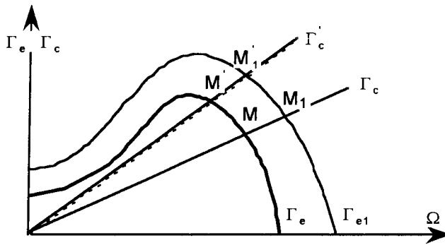
Figure 2.16: Caractéristiques de l'éolienne et de la charge - étude qualitative
