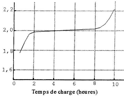
Figure 1.13a: Evolution de la tension aux bornes d'un élément en charge
