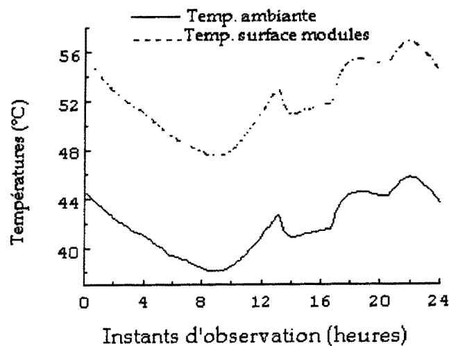
Figure 2. 6: Evolution journalière de la température ambiante et de la température à la surface des modules
