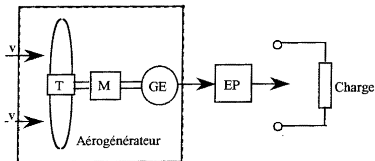
Figure 1.17: Structure de conversion de l'énergie éolienne
