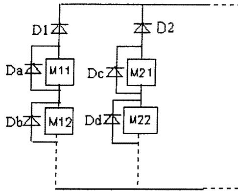
Figure 1.12: Protection par diodes en parallèle
