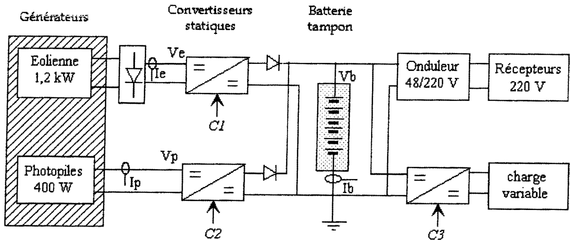
Figure 3.1: Synoptique de puissance
