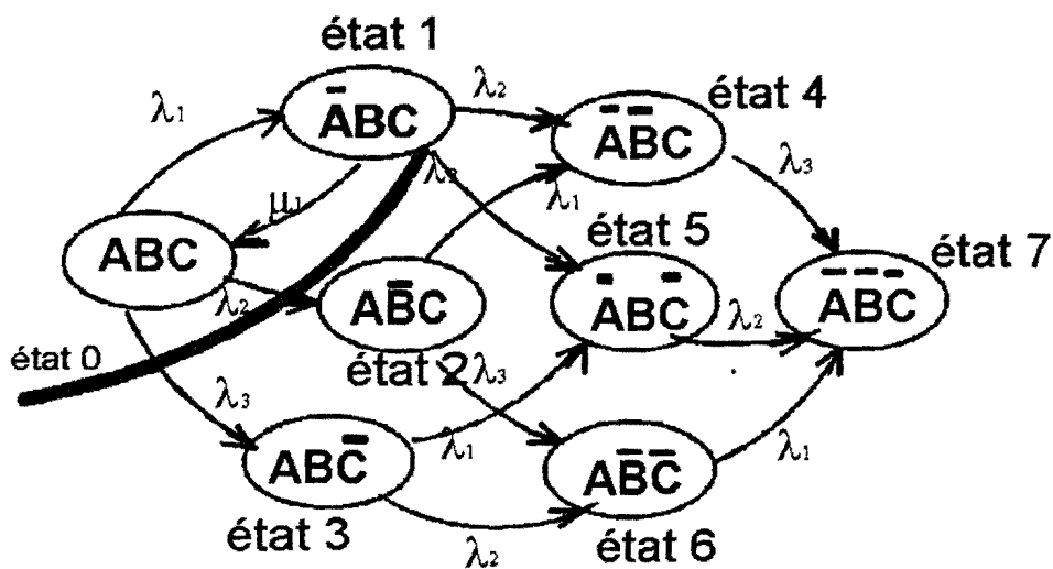
Figure 4. 11: Chaîne de Markov
