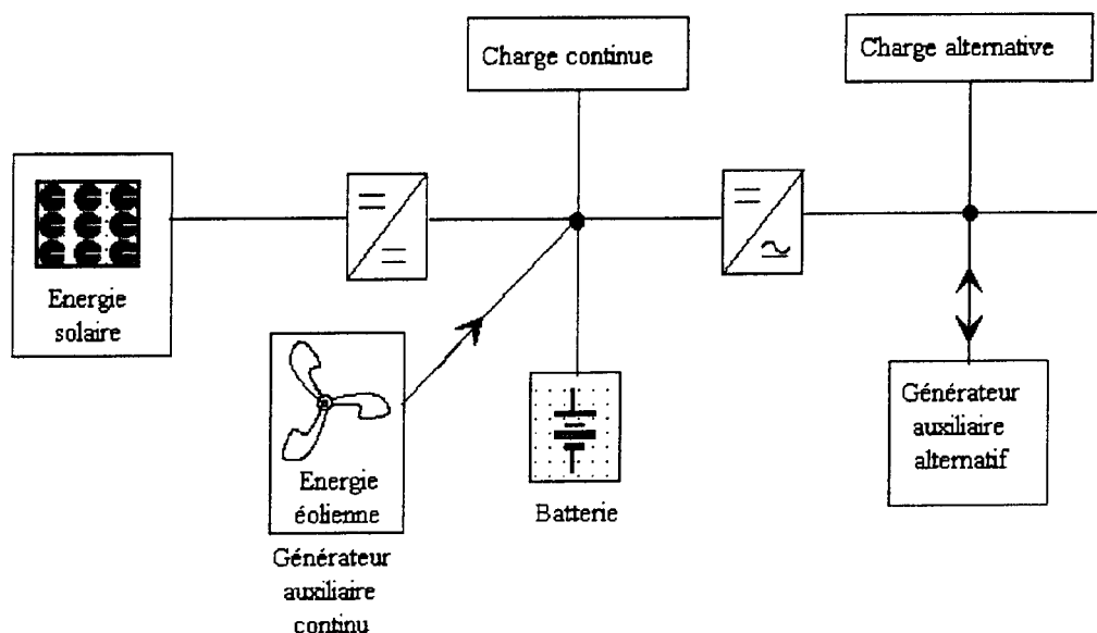
Figure 2. 1: Schéma d'un système photovoltaïque
