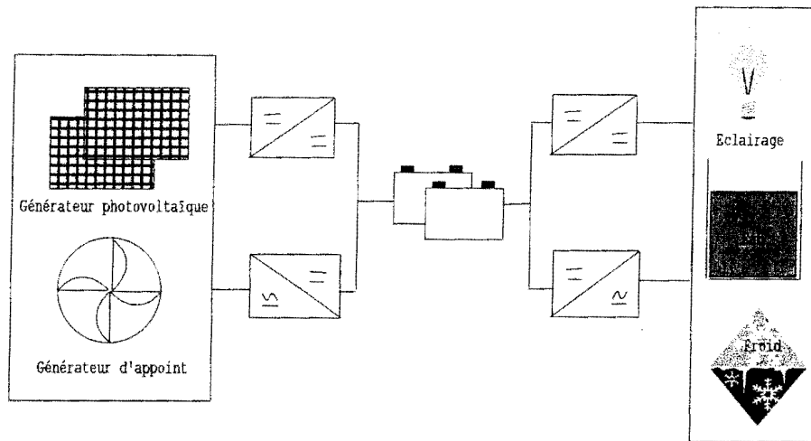
Figure 1.1: Structure des systèmes étudiés
