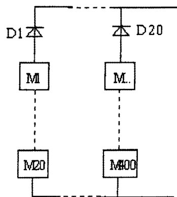
Figure 1.11: Protection par diodes en série
