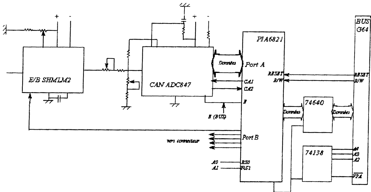
Figure 3. 8: Chaîne de conversion analogique numérique
