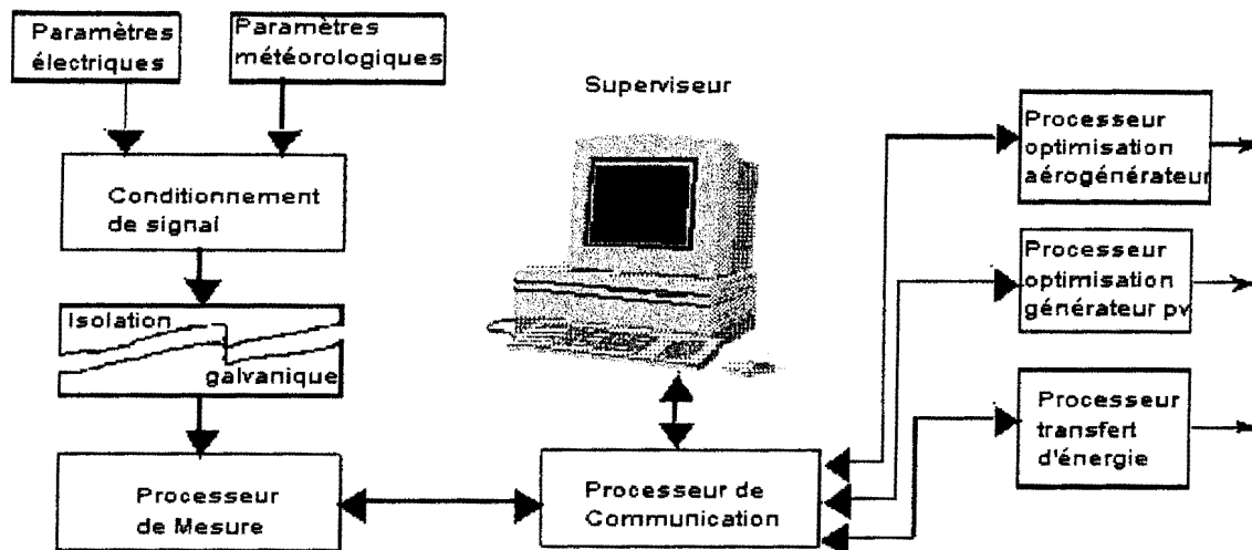
Figure 4. 4: Synoptique de la commande
