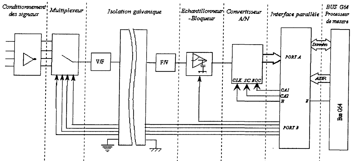
Figure 3. 6: Synoptique de la chaîne d'acquisition
