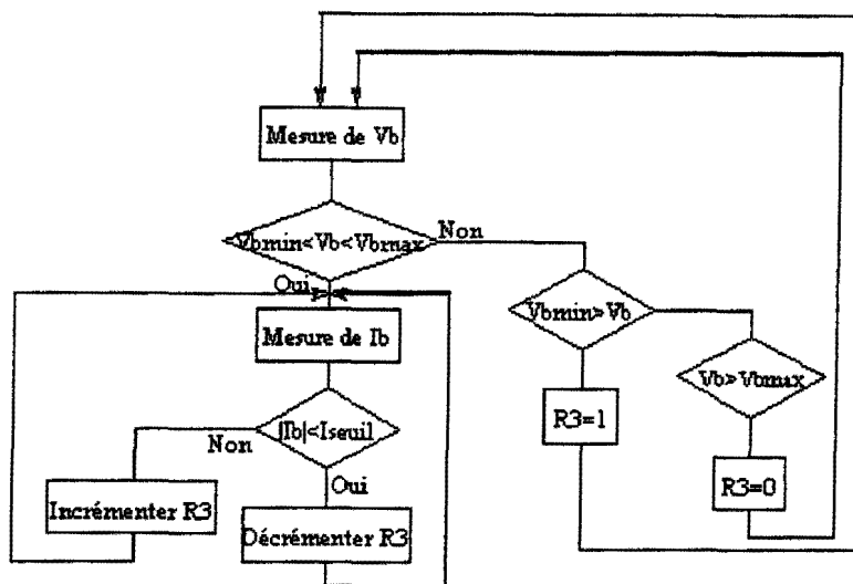
Figure 3. 14: Configuration du transfert d'énergie
