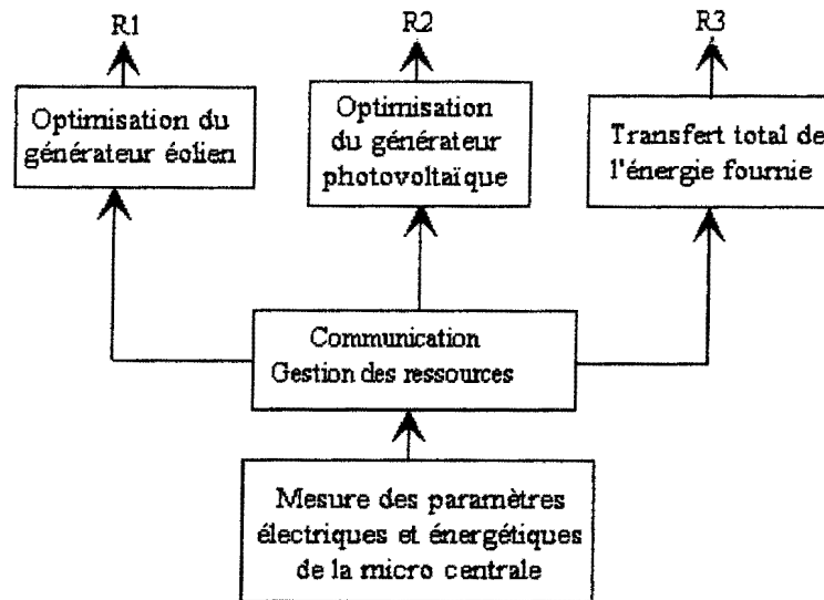
Figure 3. 3: Synoptique des tâches
