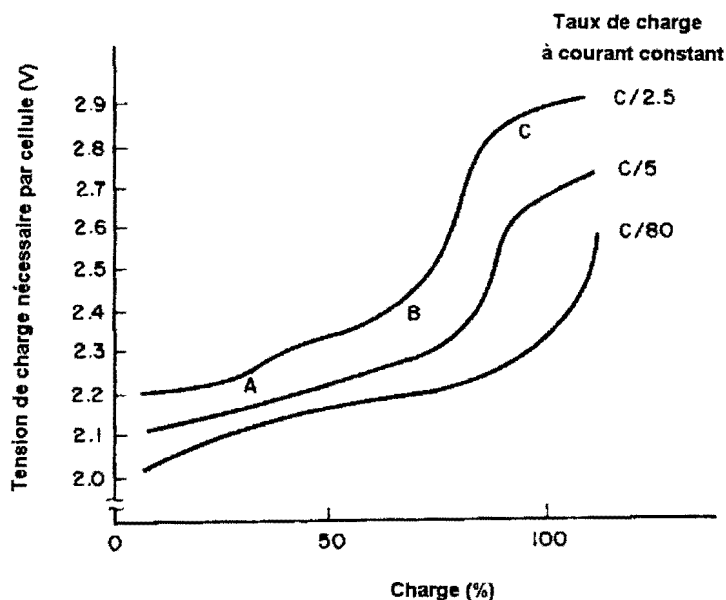
Figure 1.15 a: Tension en fonction de l'état de charge pour divers régimes de charge
