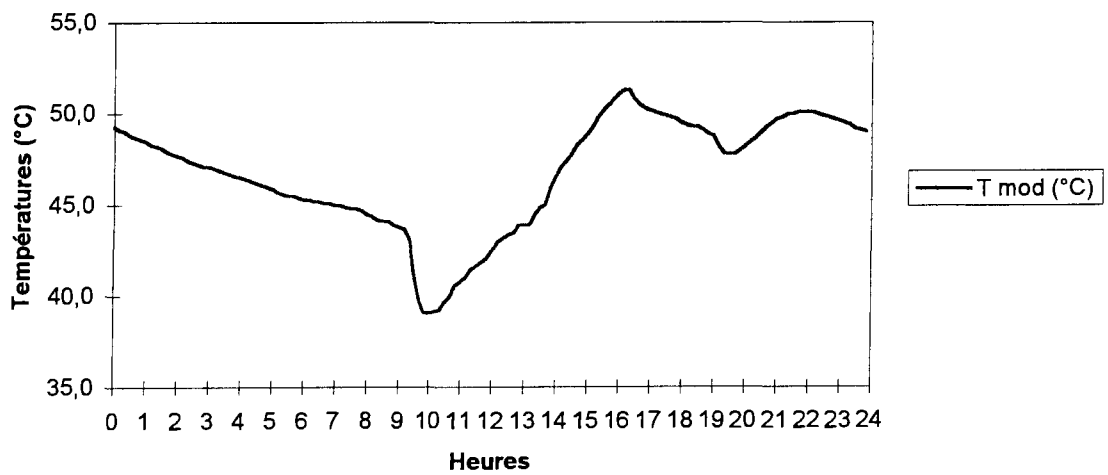
Figure 5. 15: Evolution de la température des modules
