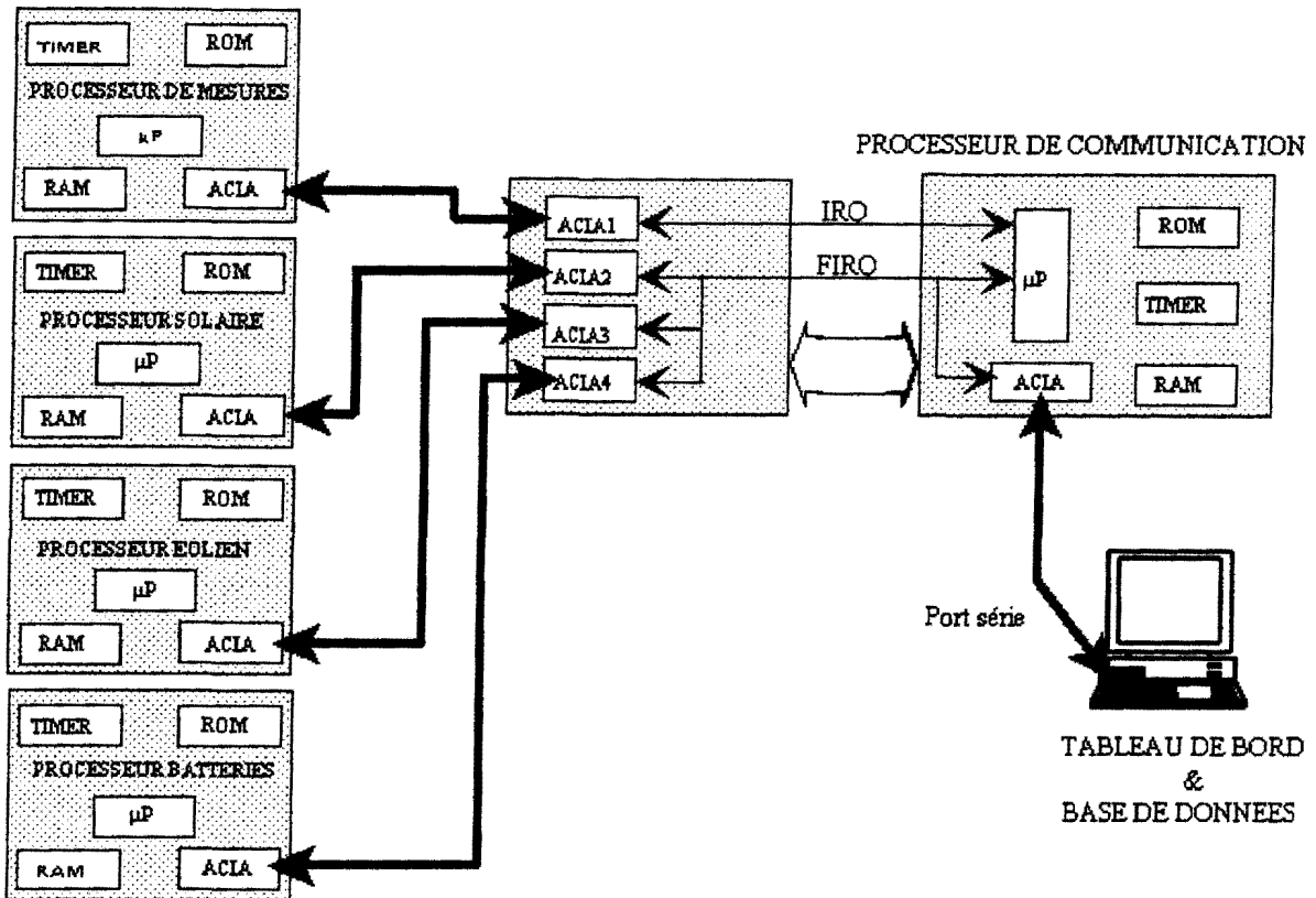
Figure 3. 4: Structure multiprocesseurs
