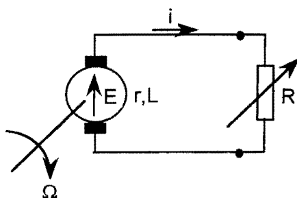
Figure 2. 15: Schéma de principe du générateur de courant continu
