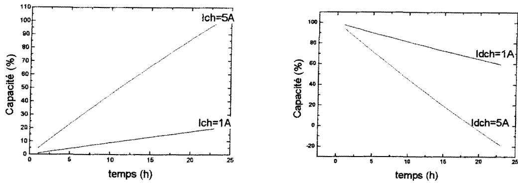
Figure 2. 10: Caractéristiques de charge et décharge en zone linéaire
