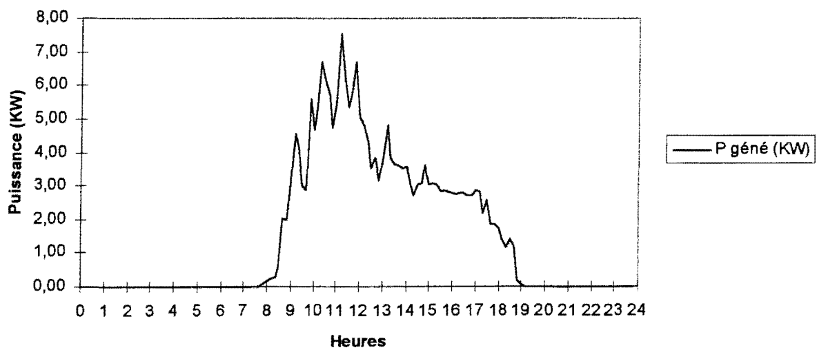
Figure 5. 16: Evolution de la puissance de sortie du générateur
