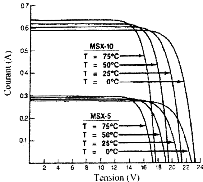
Figure 2. 5: Caractéristiques I(V) à irradiations et températures données
