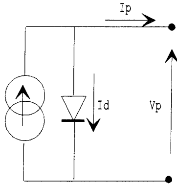
Figure 1.5: Schéma équivalent d'une cellule photovoltaïque idéale
