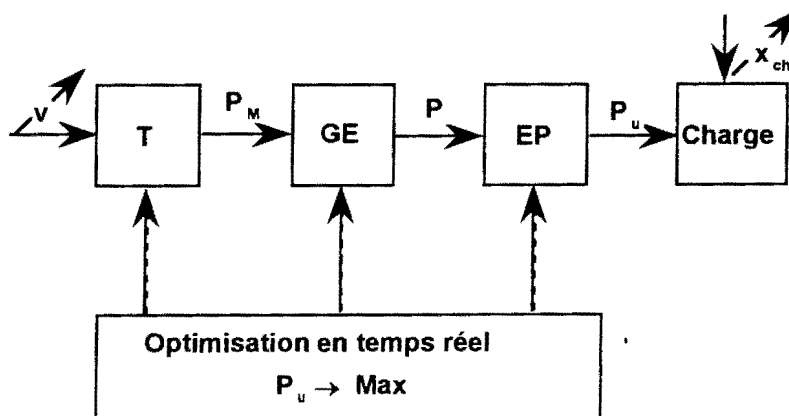
Figure 1.20: Eléments du système énergétique éolien susceptibles d'être utilisés pour l'optimisation
