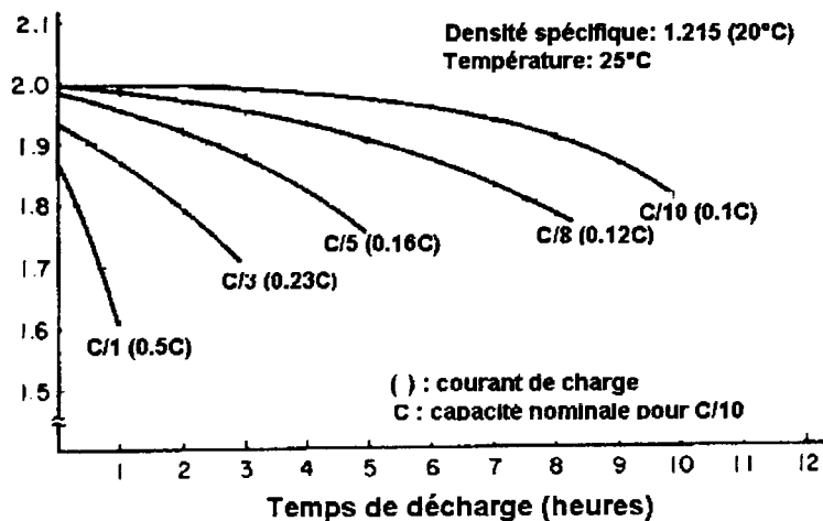
Figure 2. 11: Tension en fonction de l'état de décharge pour différents courants
