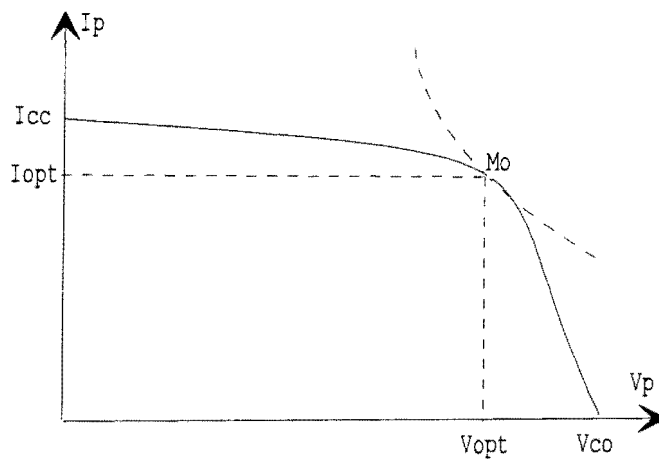
Figure 1.8: Caractéristique statique réelle d'une cellule photovoltaïque
