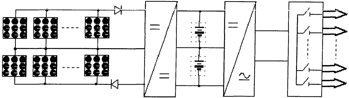
Figure 5. 1: Synoptique de la centrale de Diaoulé
