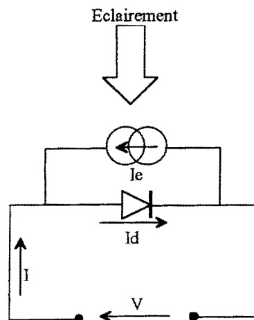
Figure 1.3: Schéma équivalent d'une cellule photovoltaïque soumise à un éclairement
