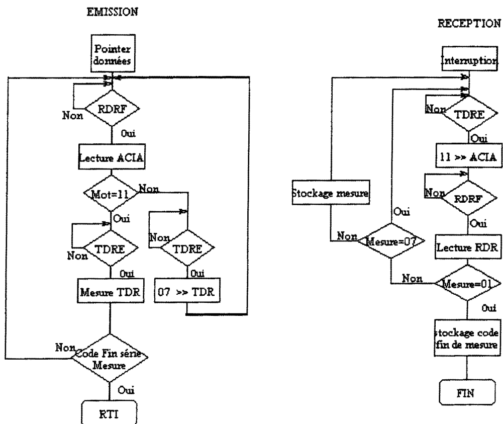
Figure 3. 12: Organigramme de la procédure de communication
