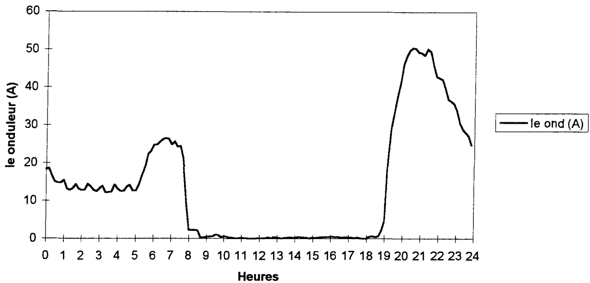
Figure 5. 20: Evolution du courant d'entrée de l'onduleur
