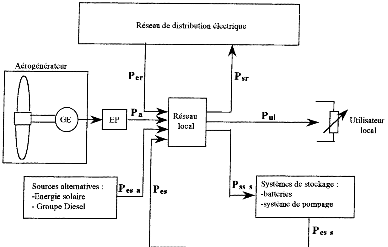
Figure 1.18: Schéma général de conversion de l'énergie éolienne
