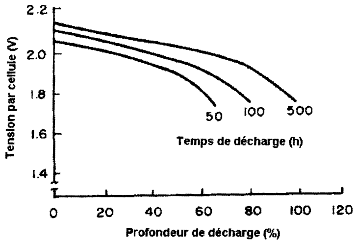
Figure 1.14: Tension aux bornes d'un élément en fonction de la profondeur de décharge avec le temps de décharge en paramètre
