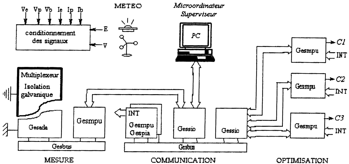
Figure 3.2: Synoptique de commande
