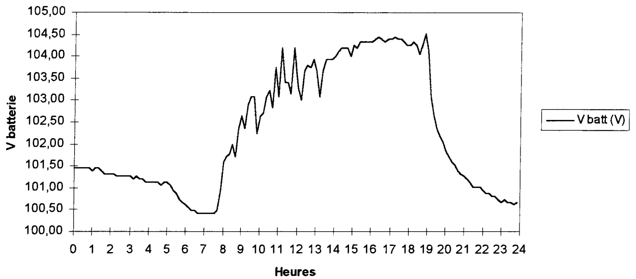
Figure 5. 21: Evolution de la tension aux bornes des batteries
