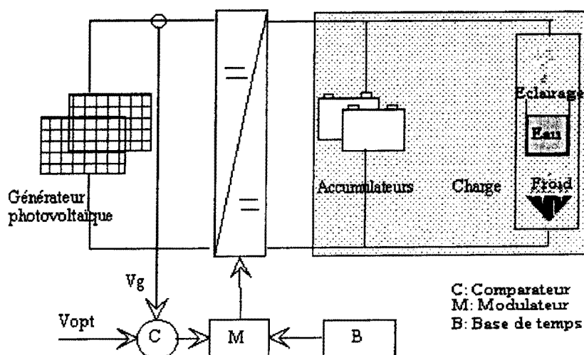
Figure 1.22: Techniques de poursuite du point de fonctionnement optimal
