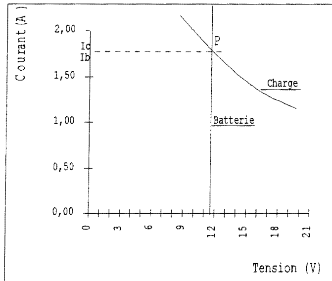
Figure 1.30: Représentation graphique du point de fonctionnement (Batteries + Charge)
