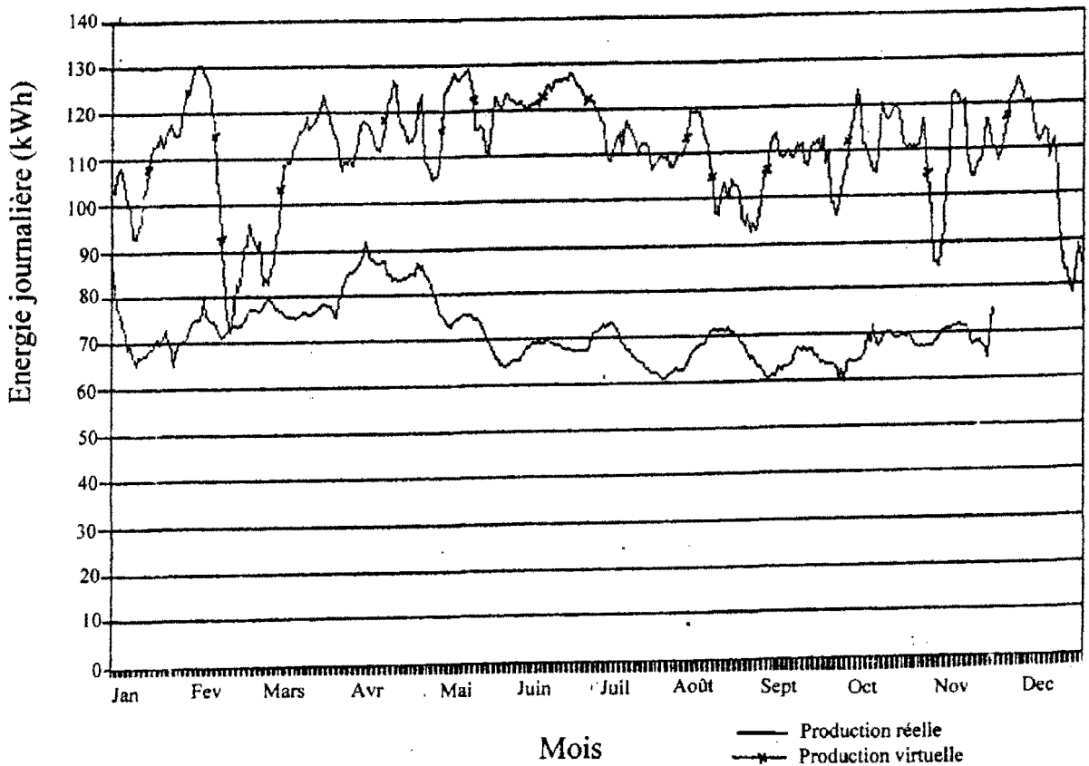
Figure 5. 8: Production sur consommation Diaoulé - 1995
