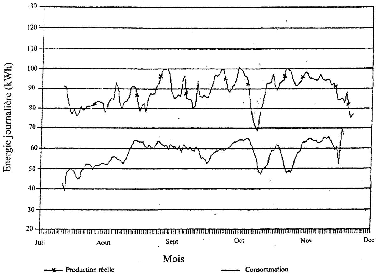
Figure 5. 6: Production sur consommation Ndiébel - Juillet/Novembre 1995
