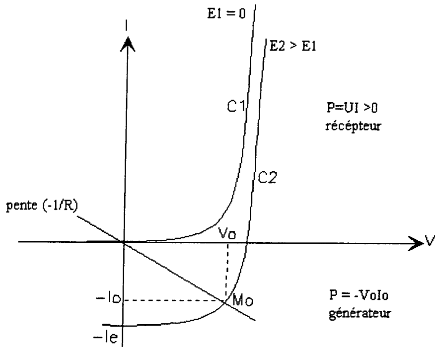
Figure 1.4: Caractéristique I = f(V) .
