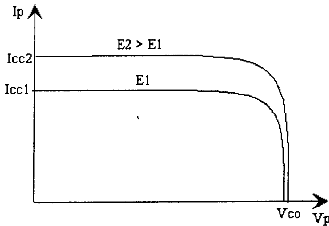
Figure 1.6: Caractéristique I_p = f(V_p) d'une cellule idéale
