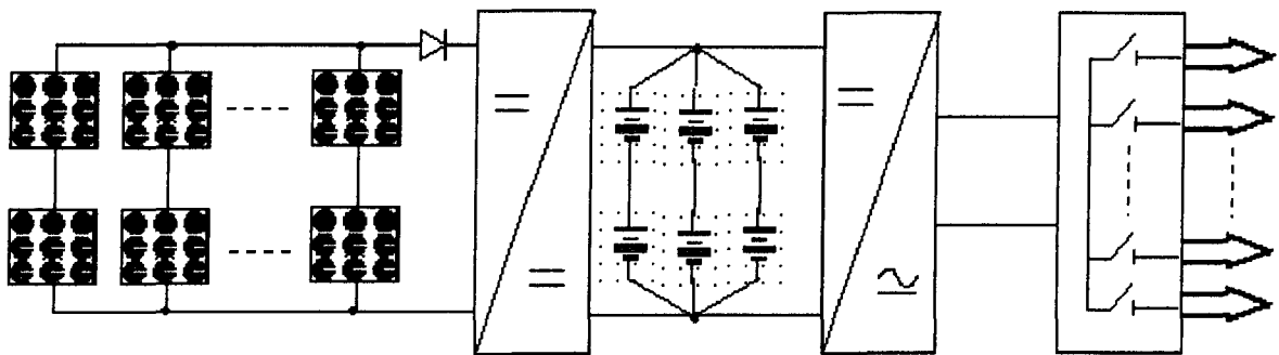
Figure 5. 2: Synoptique de la centrale de Ndiébel
