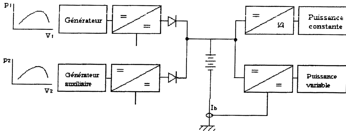
Figure 1.21: Couplage multigénérateurs par diodes et batterie tampon
