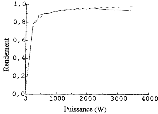
Figure 2. 9: Caractéristiques de rendement
