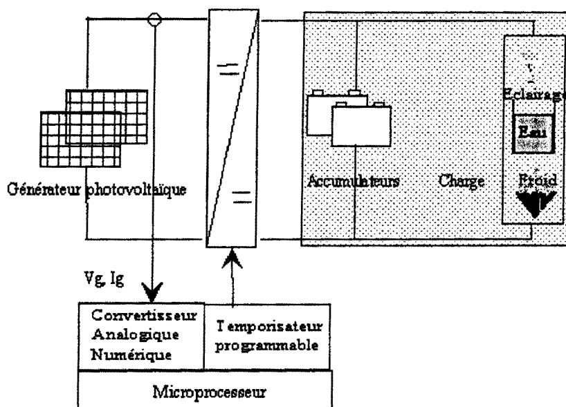
Figure 1.23: Contrôle numérique du point de fonctionnement optimal
