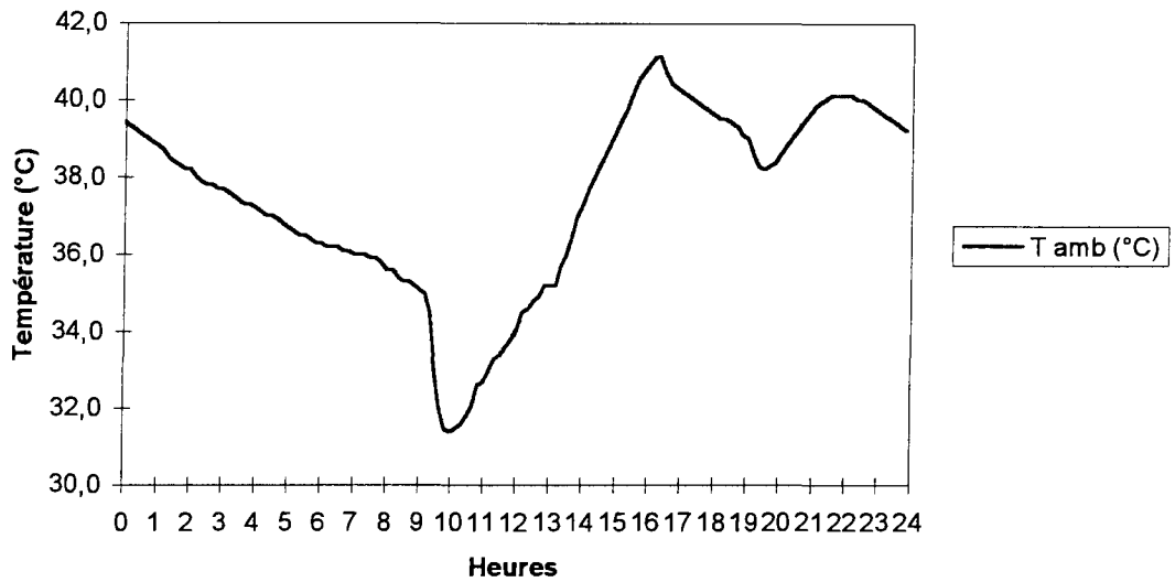
Figure 5. 14: Evolution de la température ambiante
