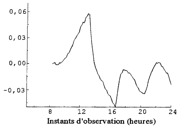
Figure 2. 4: Ecart relatif entre températures ambiantes mesurée et simulée
