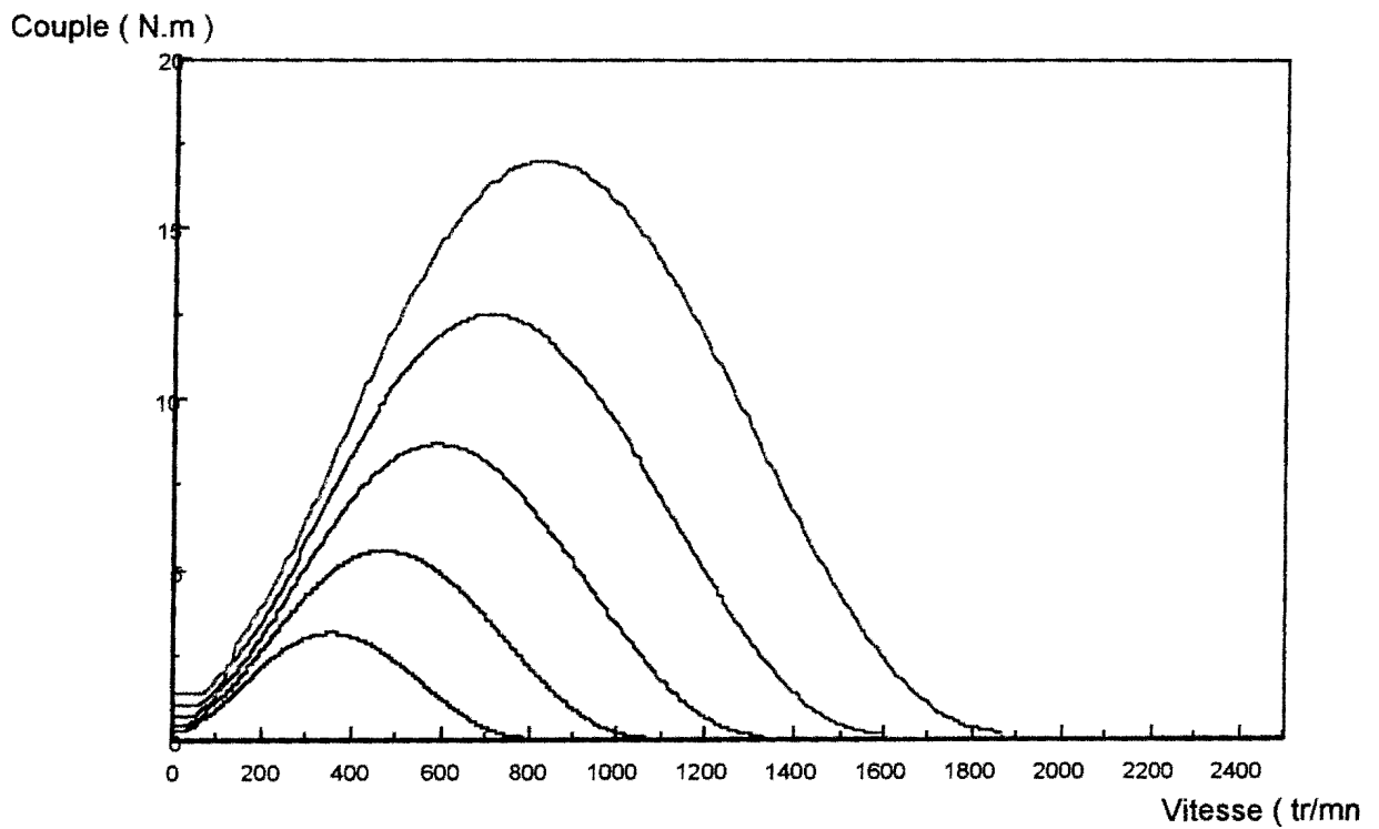
Figure 2. 13: Couple éolien en fonction de la vitesse sur l'axe
