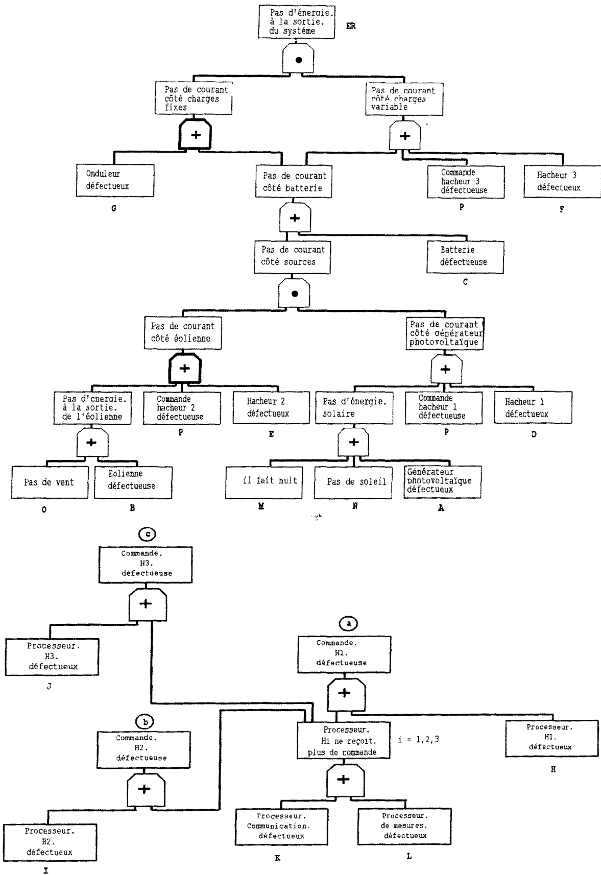
Figure 4. 9: Analyse quantitative par Arbre des causes
