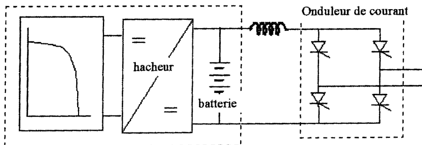
Figure 1.25: Synoptique de principe de l'onduleur de courant
