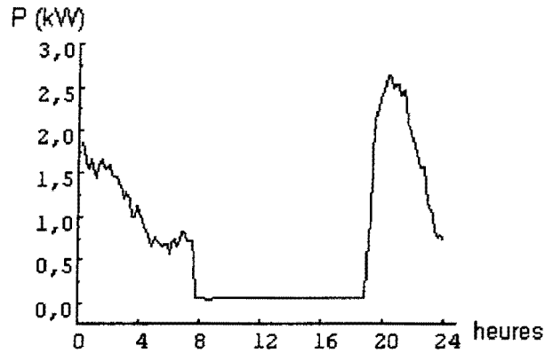
Figure 2. 21: Profil de consommation
