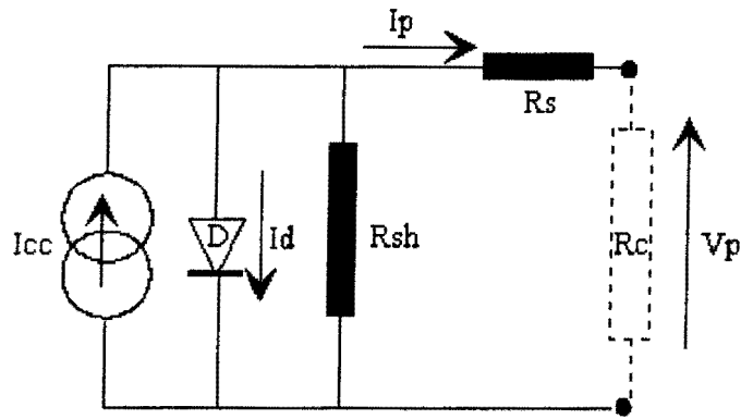
Figure 1.7: Schéma équivalent d'une cellule photovoltaïque réelle
