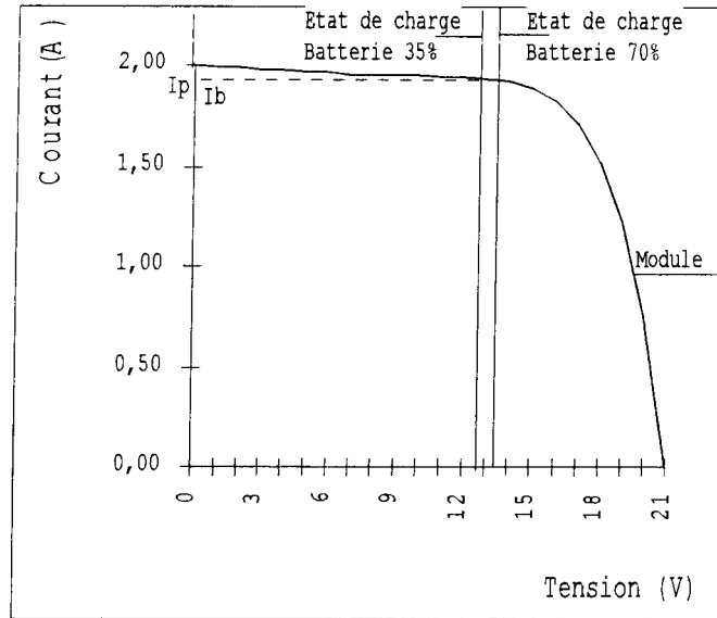
Figure 1.31: Représentation graphique du point de fonctionnement (GPV + Batteries)
