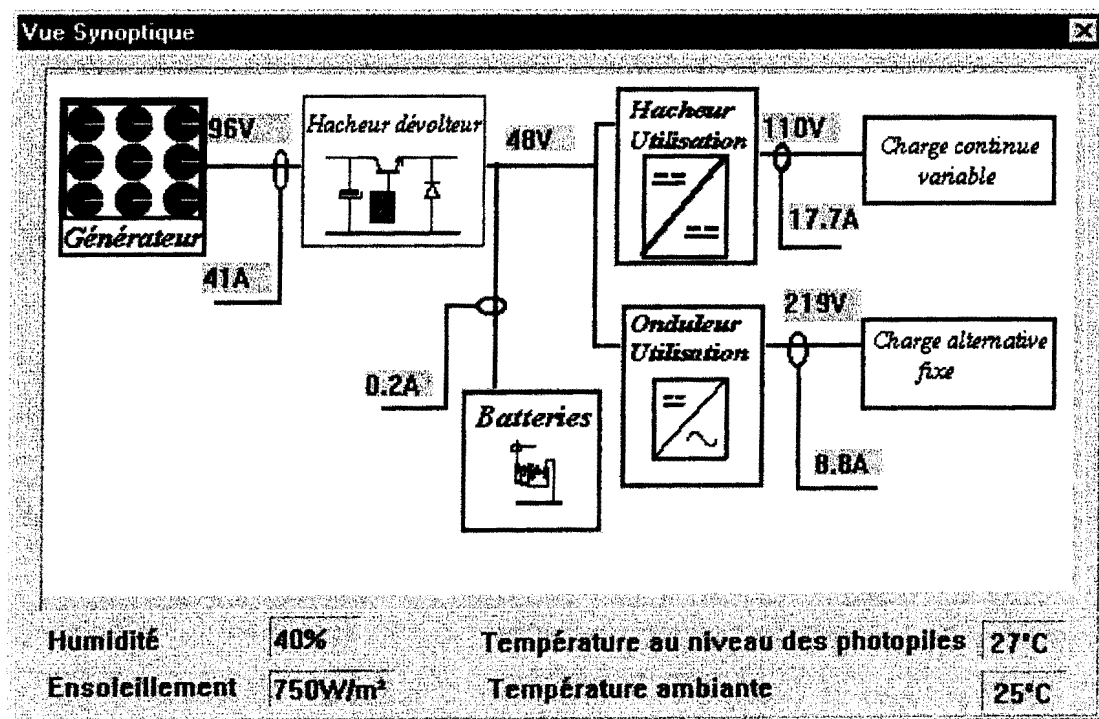
Figure 3. 17: Vue synoptique de l'application spécifique de supervision
