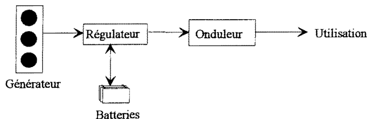
Figure 5. 23: Architecture d'un système photovoltaïque décentralisé type.
