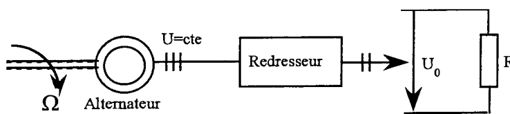
Figure 2.17: Alternateur connecté à un pont triphasé
