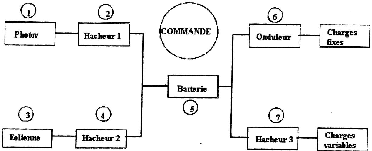
Figure 4. 5: Agencement du sous-système de puissance
