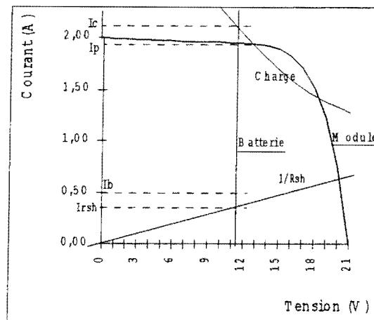
Figure 1.36: Régulation par dérivation du courant
