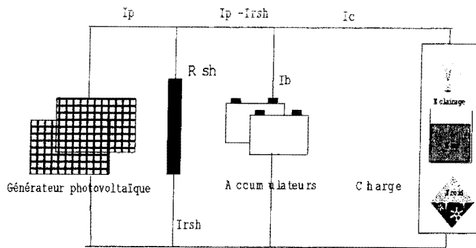
Figure 1.35: Schéma simplifié de la configuration
