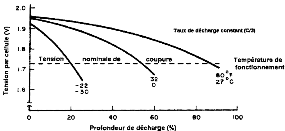
Figure 1.15 b: Tension de décharge en fonction de la température
