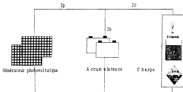
Figure 1.27: Schéma de principe du système
