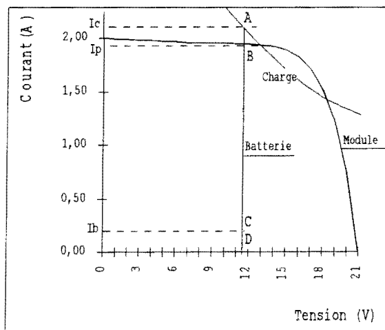
Figure 1.29: Représentation graphique du point de fonctionnement (GPV + Batteries + Charge)
