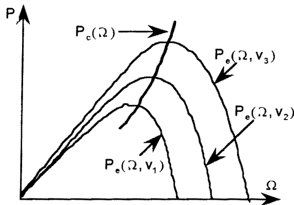
Figure 1.19: Conversion optimale de l'énergie éolienne
