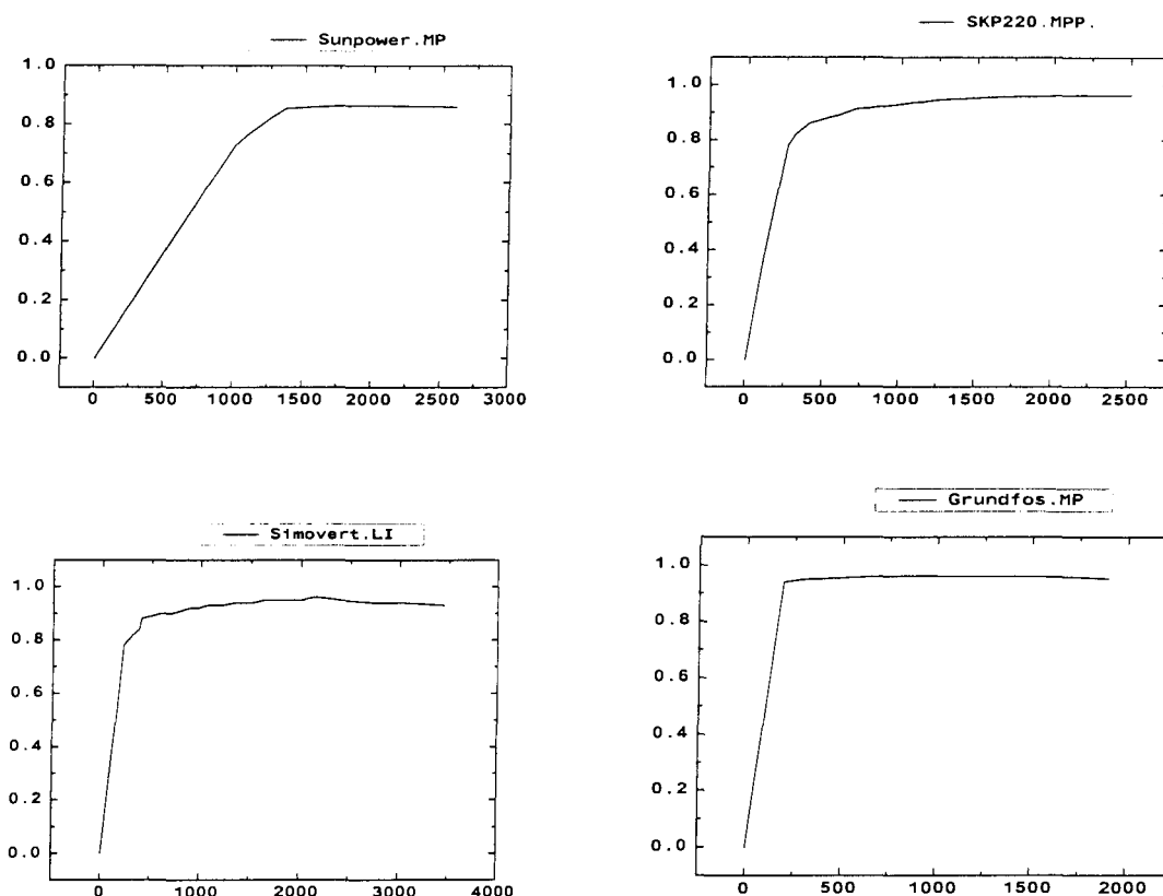
Figure 1.24: Exemples de rendement selon quatre constructeurs
