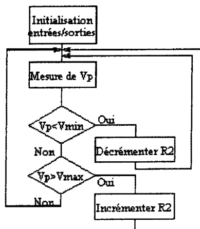
Figure 3. 13: Optimisation du générateur photovoltaïque
