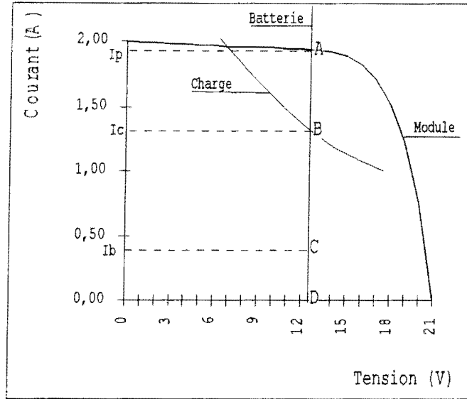
Figure 1.28: Représentation graphique du point de fonctionnement (GPV + Batterie + Charge)
