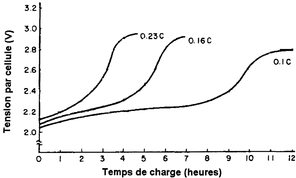
Figure 2. 12: Tension en fonction de l'état de charge pour différents courants
