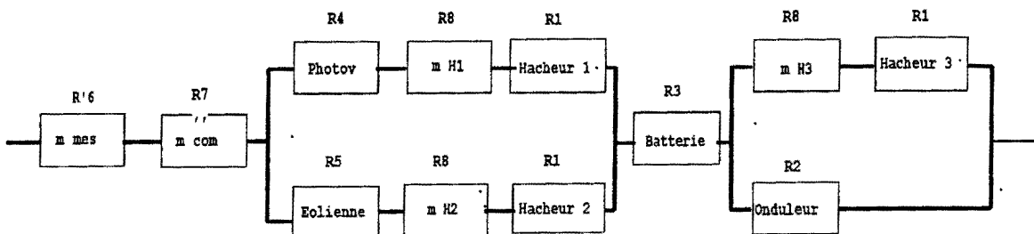
Figure 4. 7: Bloc diagramme multiprocesseur
