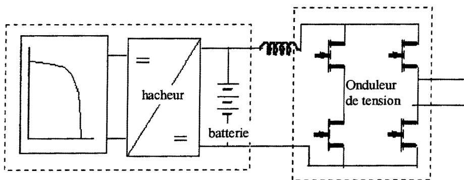
Figure 1.26: Synoptique de principe de l'onduleur de tension
