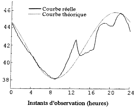
Figure 2. 3: Caractéristiques comparées de température
