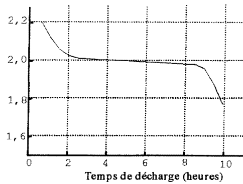
Figure 1.13b: Evolution de la tension aux bornes d'un élément en décharge
