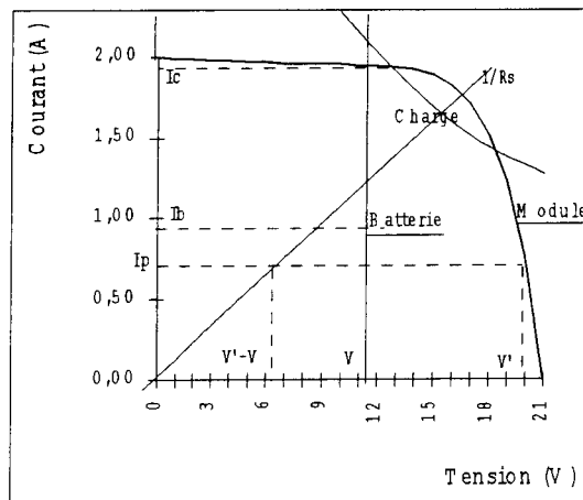
Figure 1.34: Adjonction d'une résistance série
