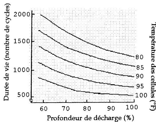
Figure 1.16: Effet de la profondeur de décharge et de la température sur la durée de vie
