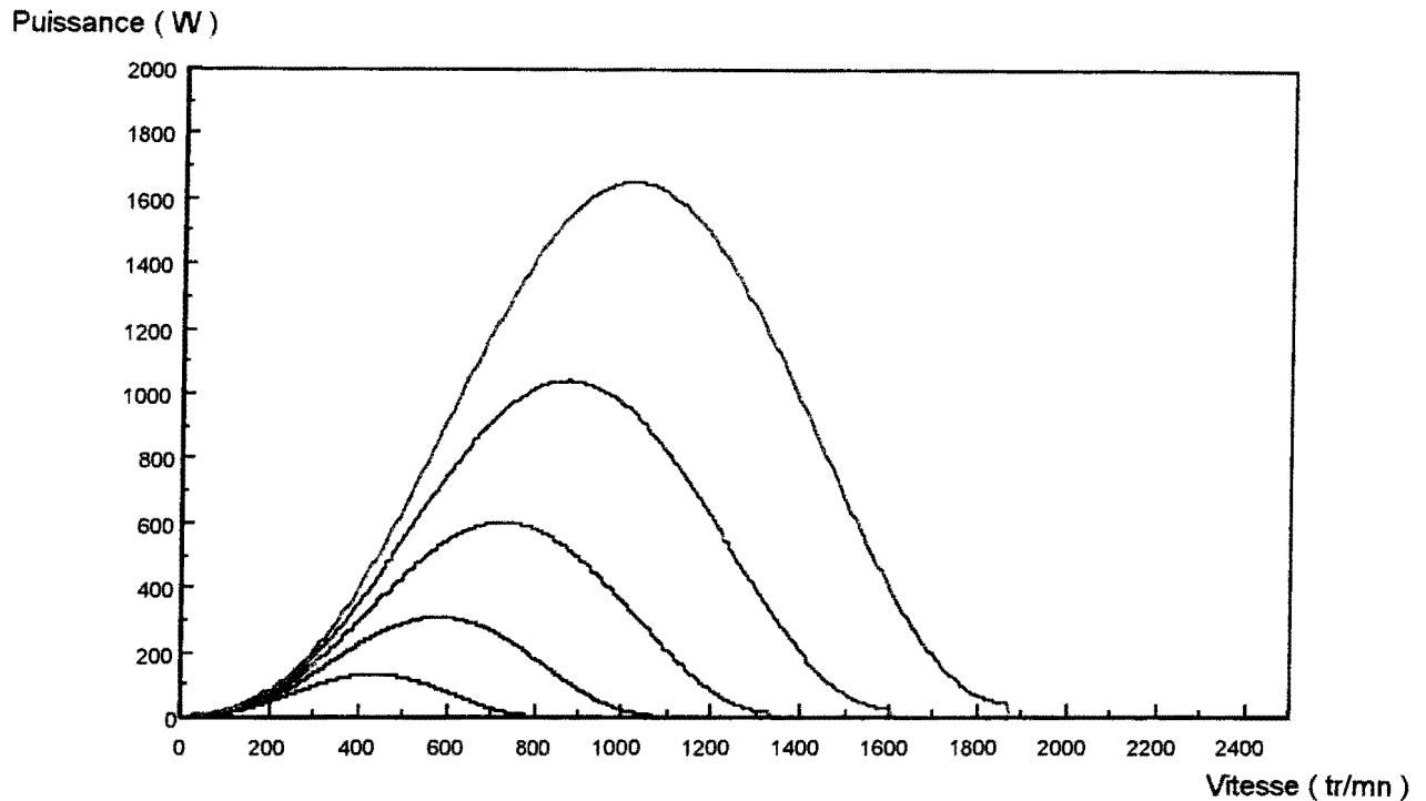
Figure 2. 14: Puissance éolienne en fonction de la vitesse sur l'axe
