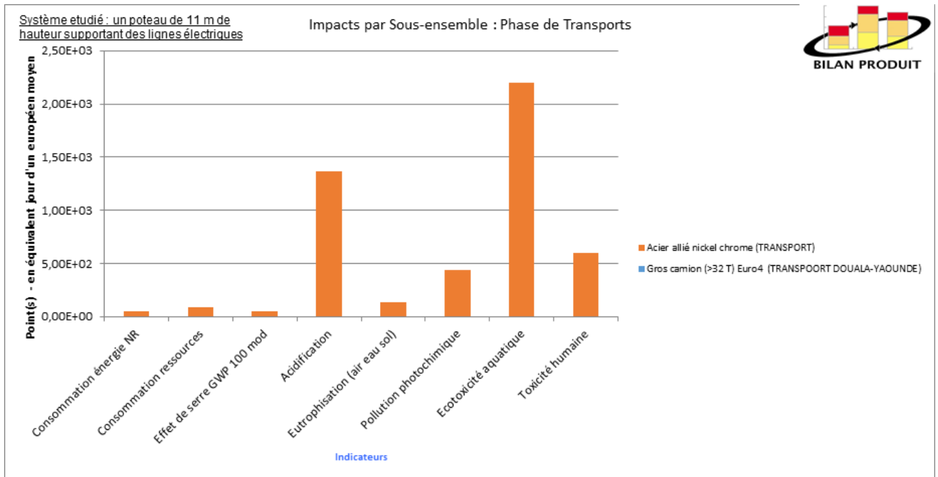
FIGURE 3.6 – Impact par sous ensemble-Phase de transport des PEA
