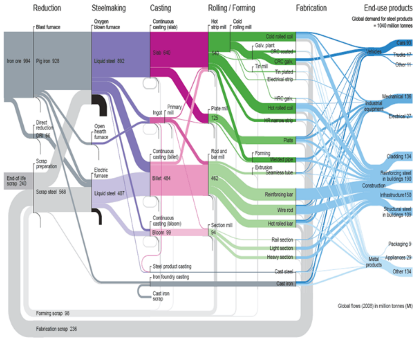
FIGURE 2.11 – Analyse de l'inventaire de cycle de vie de poteaux en acier (PNUE,1986)
