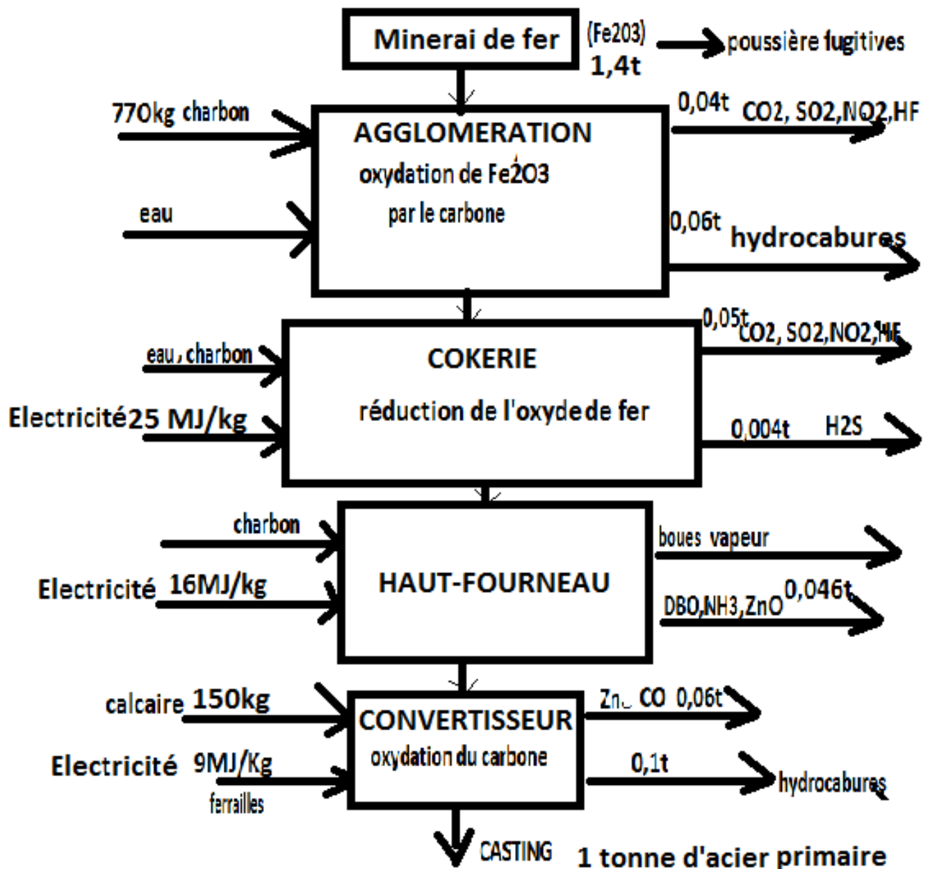
FIGURE 2.7 – production primaire d'une tonne l'acier à partir de minerai de fer
