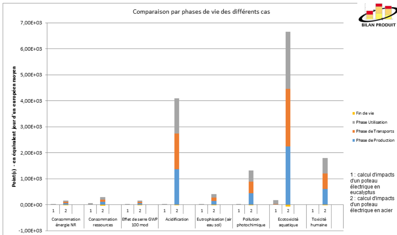
FIGURE 3.11 – Comparaison par phase de vie des différents cas
