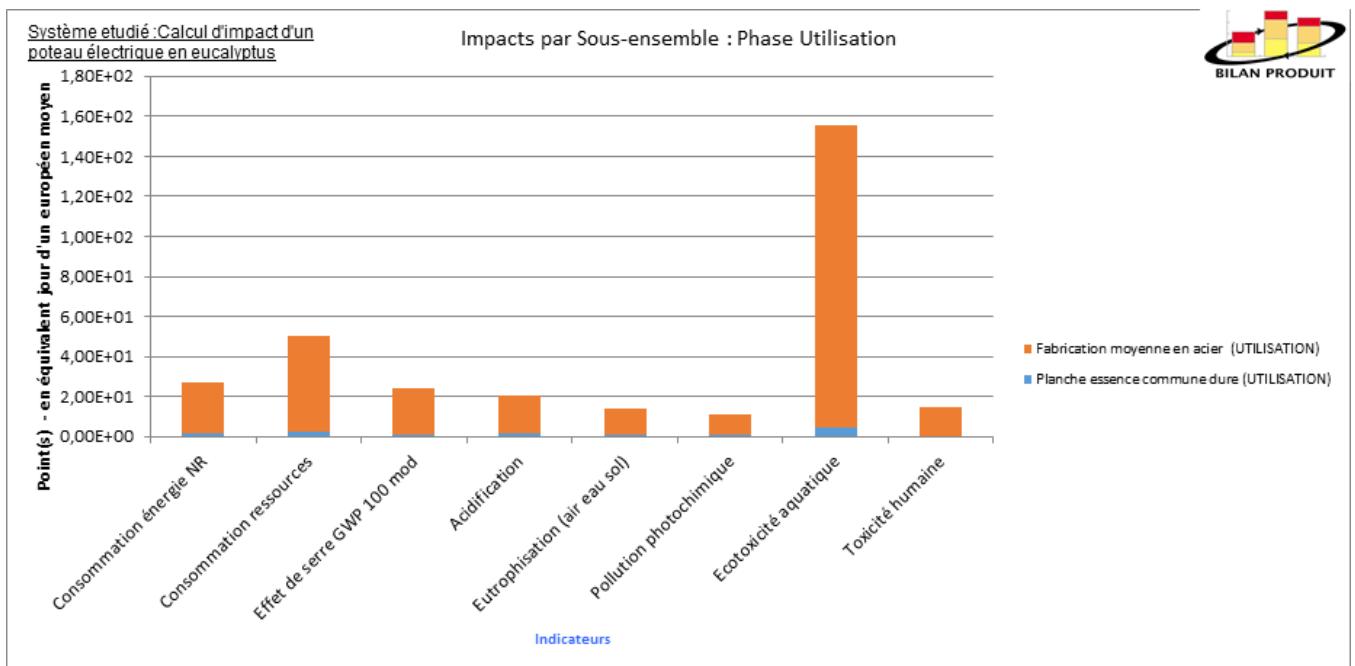
FIGURE 3.3 – Impact par sous ensemble-Phase d'utilisation des PEE
