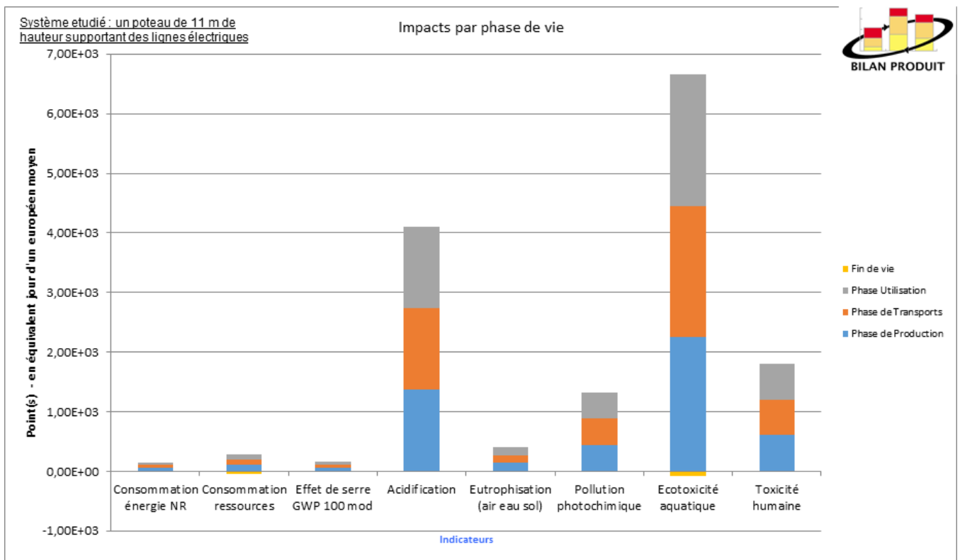
FIGURE 3.9 – Impact par phase de vie des poteaux électriques en Acier
