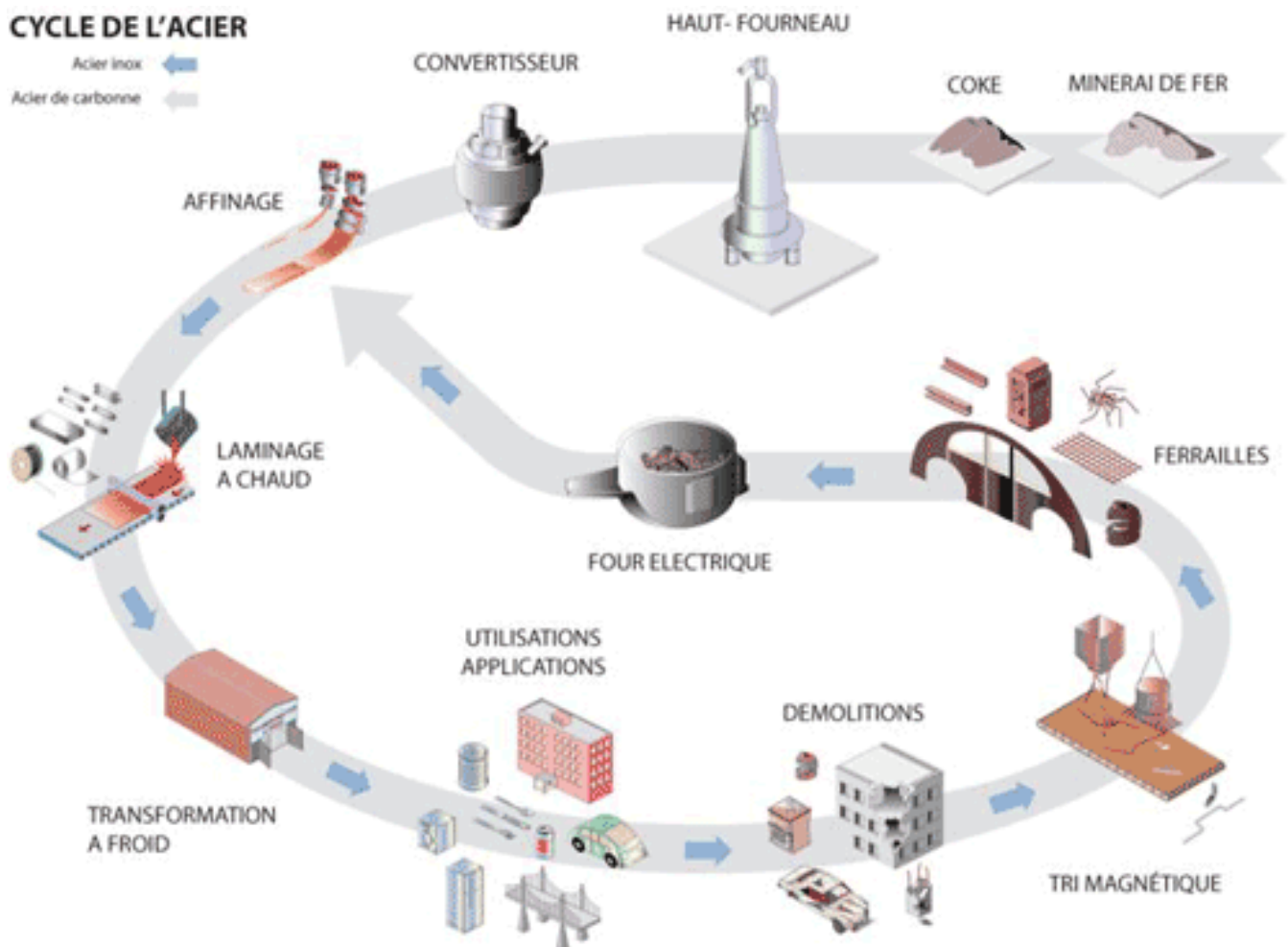
FIGURE 1.5 – Cycle de production de l'acier avec extraction du fer
