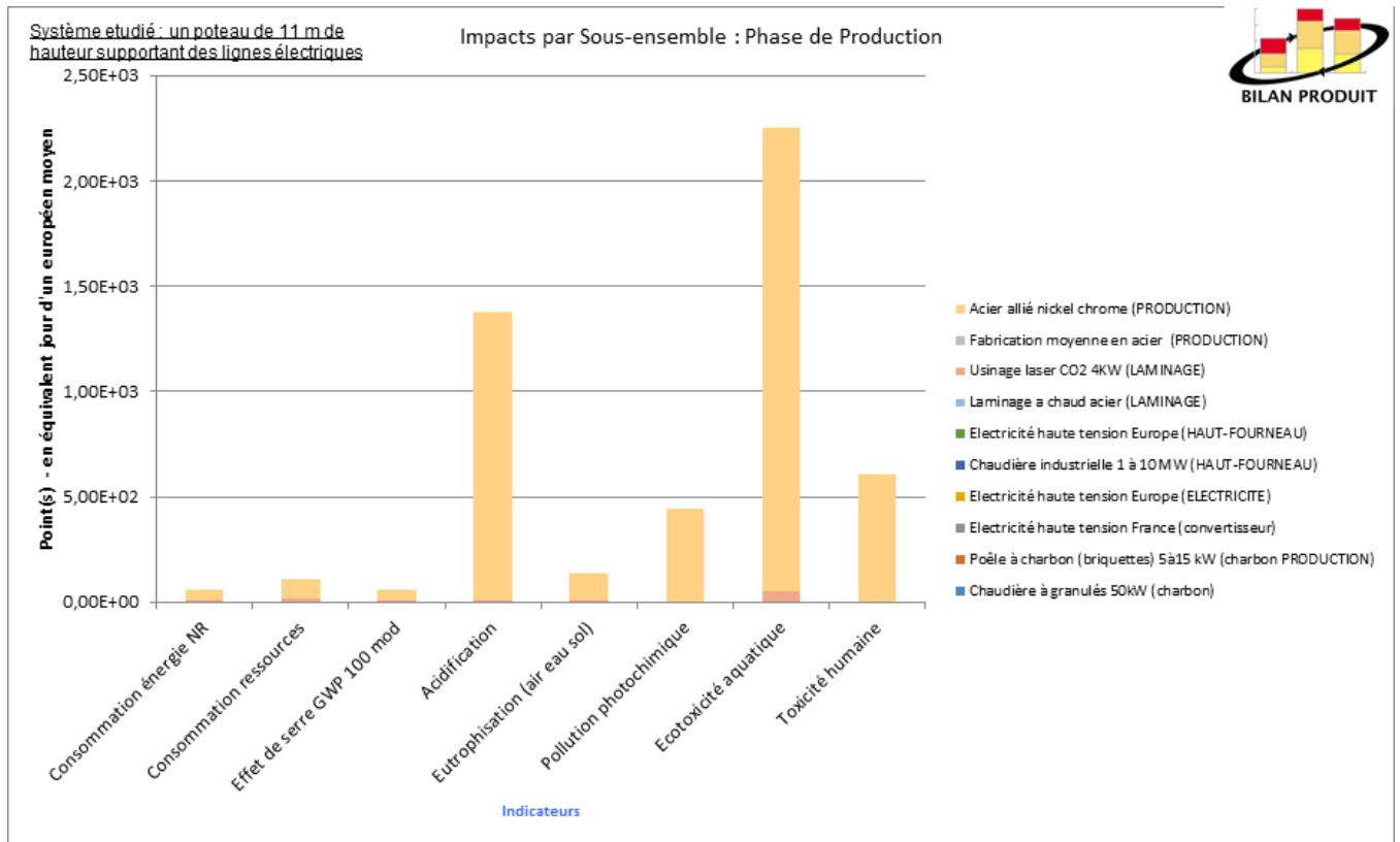
FIGURE 3.5 – Impact par sous ensemble-Phase de production des PEA
