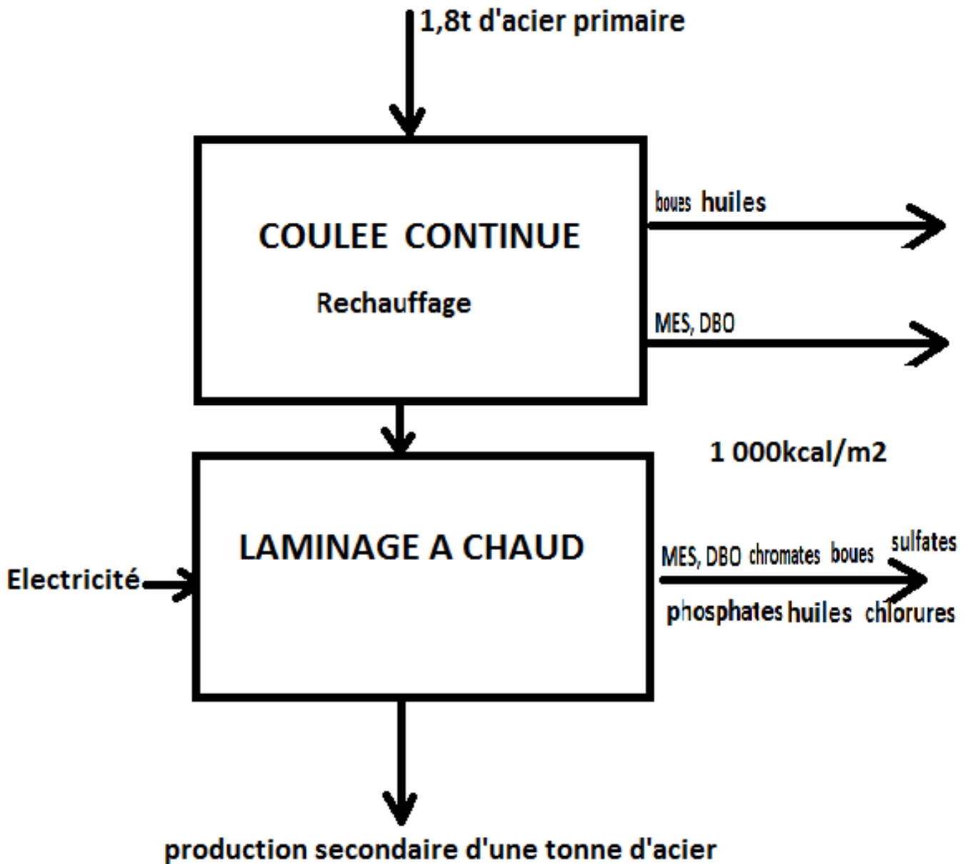
FIGURE 2.8 – production secondaire d’une tonne d’acier
