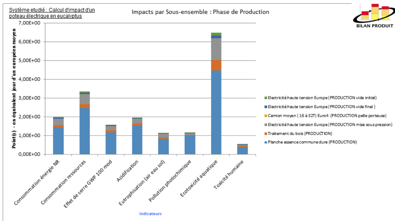
FIGURE 3.1 – Impact par sous ensemble-Phase de production des PEE
