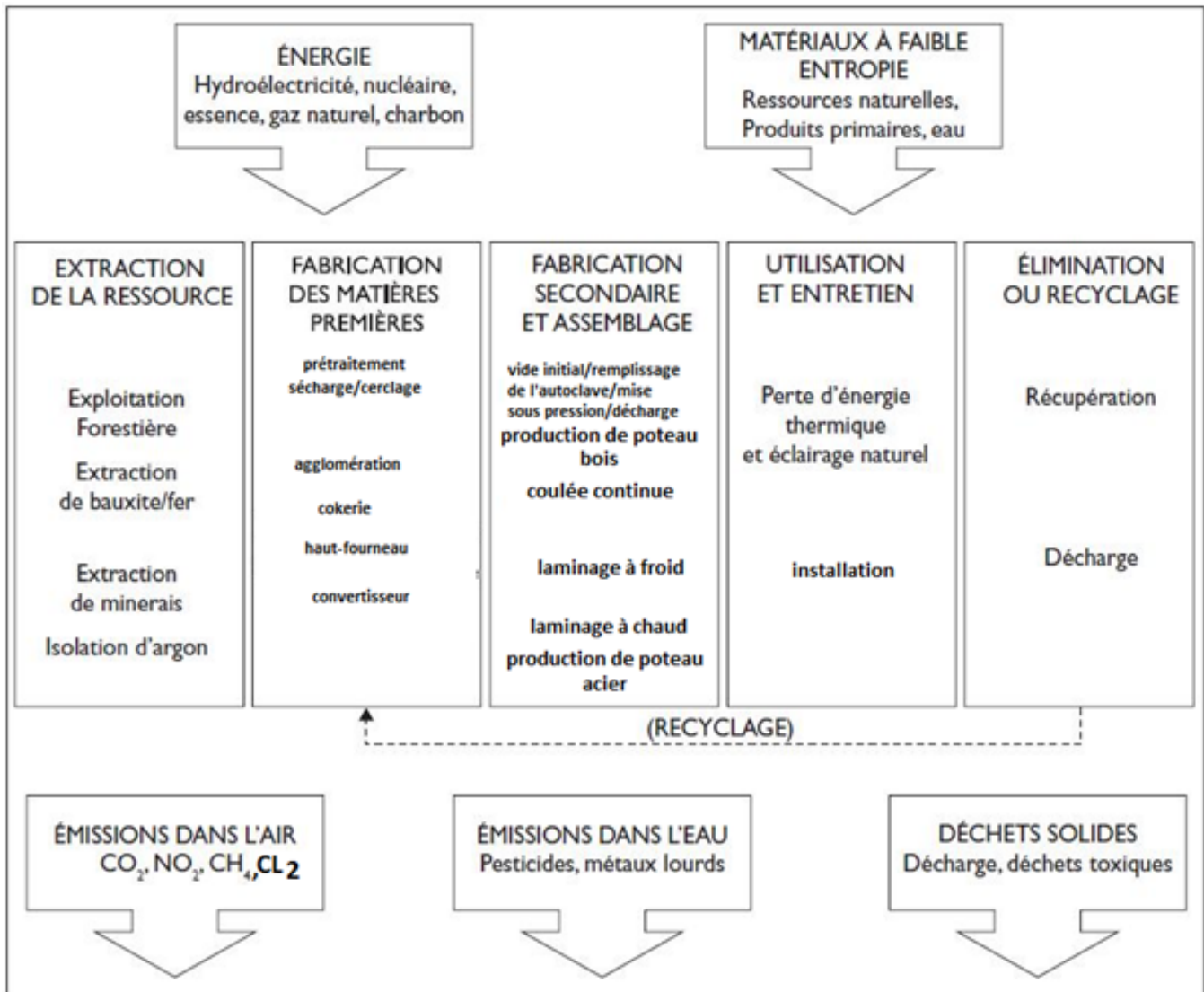
FIGURE 2.9 – Récapitulatif des deux cycles de vie
