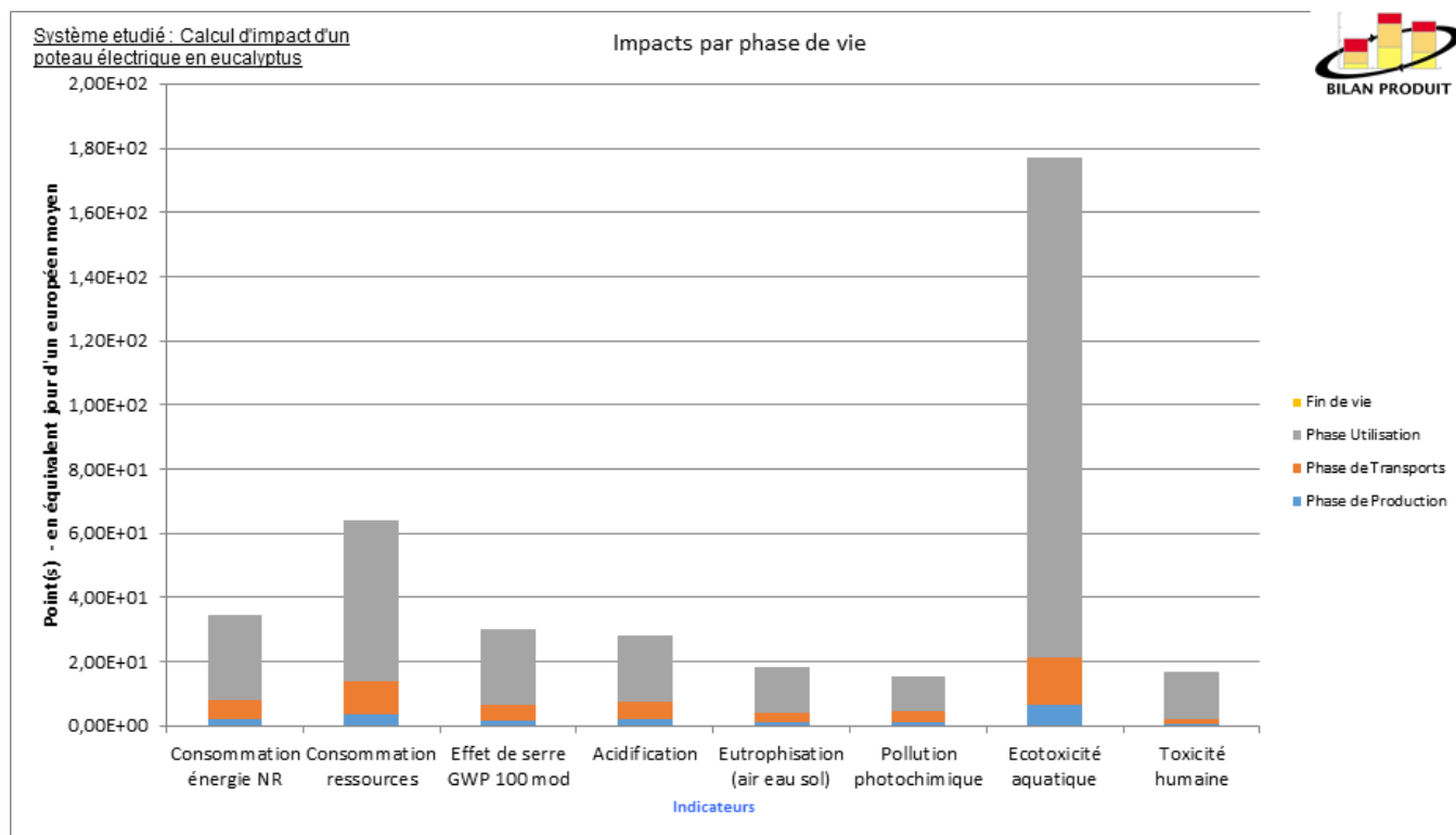
FIGURE 3.4 – Impact par phase de vie des poteaux électriques en eucalyptus
