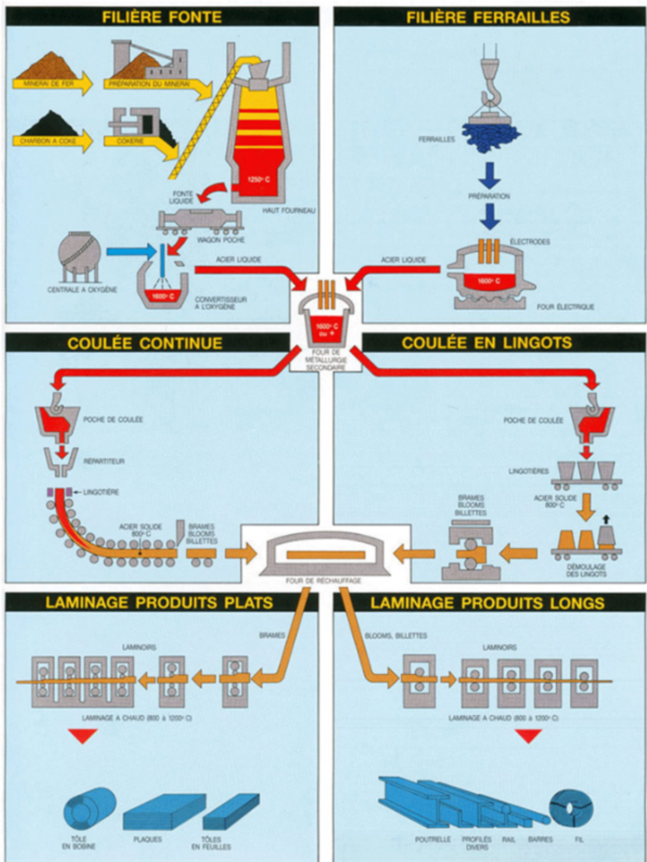
FIGURE 2.6 – cycle de production du poteau d'acier
